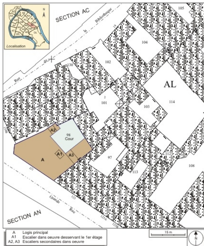
Plan masse et de situation. Extrait du plan cadastral, 1974, section AL. 25, Besançon, 121 Grande Rue, lieudit : îlot Saint-Maurice
