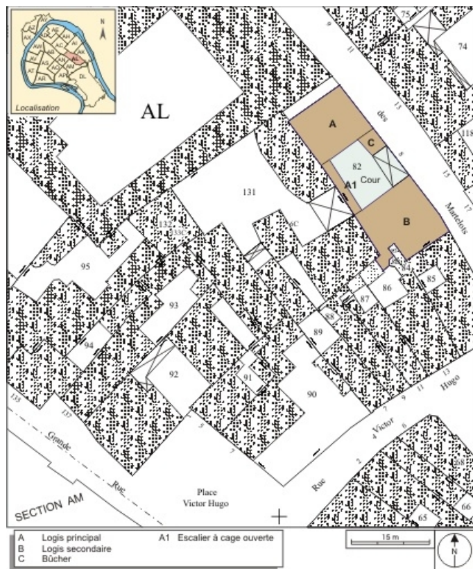
Plan masse et de situation. Extrait du plan cadastral, 1974, section AL. 25, Besançon, 8 rue des Martelots, lieudit : îlot Saint-Maurice
