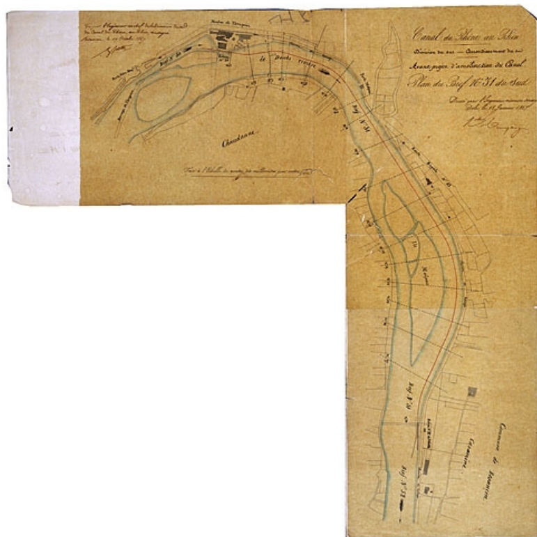
Avant-projet d'amélioration du canal. Plan du bief n° 51 du sud [du moulin de Tarragnoz à Velotte], 1847. 25, Besançon
