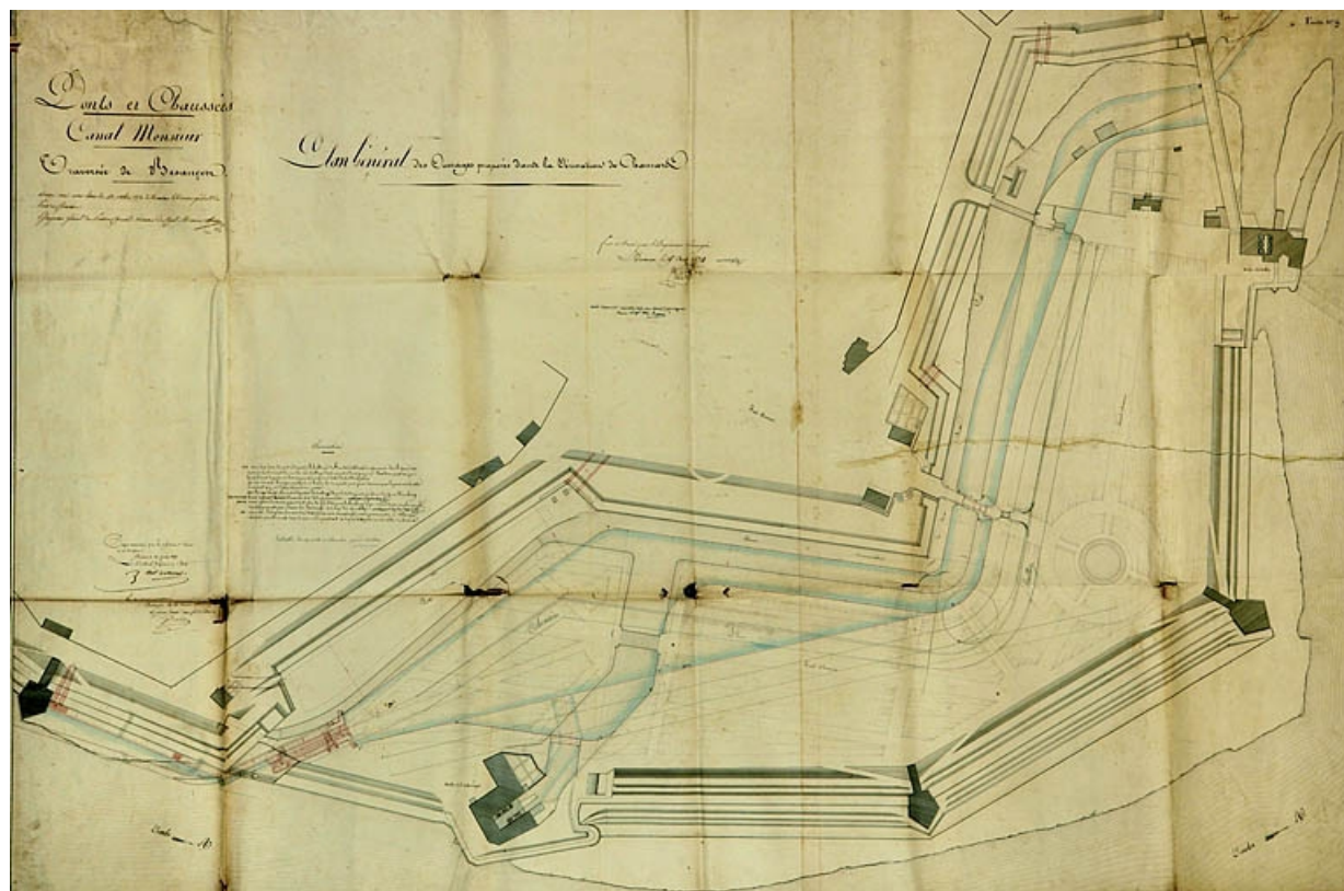
Plan général des ouvrages proposés dans la dérivation de Chamars, 1824. 25, Besançon
