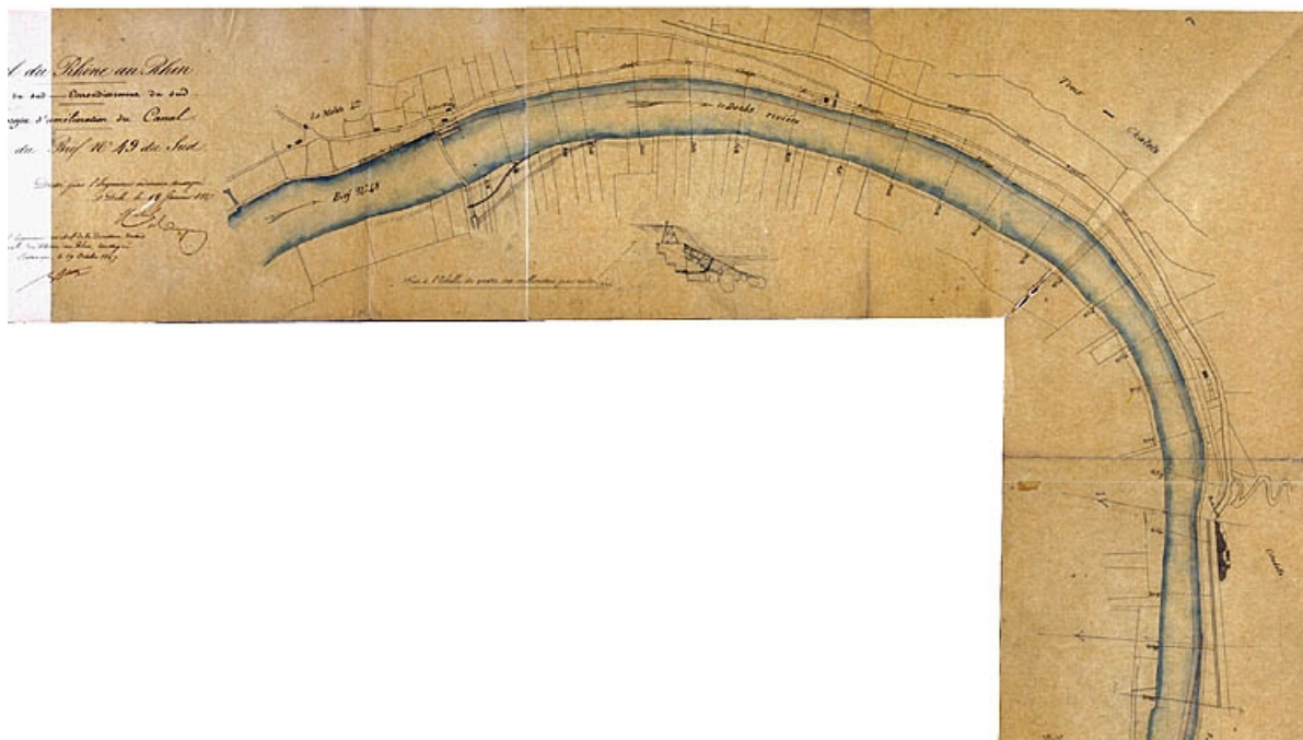
Avant-projet d'amélioration du canal. Plan du bief n° 49 du sud [détail : de la Malate à la Porte Taillée], 1847. 25, Besançon
