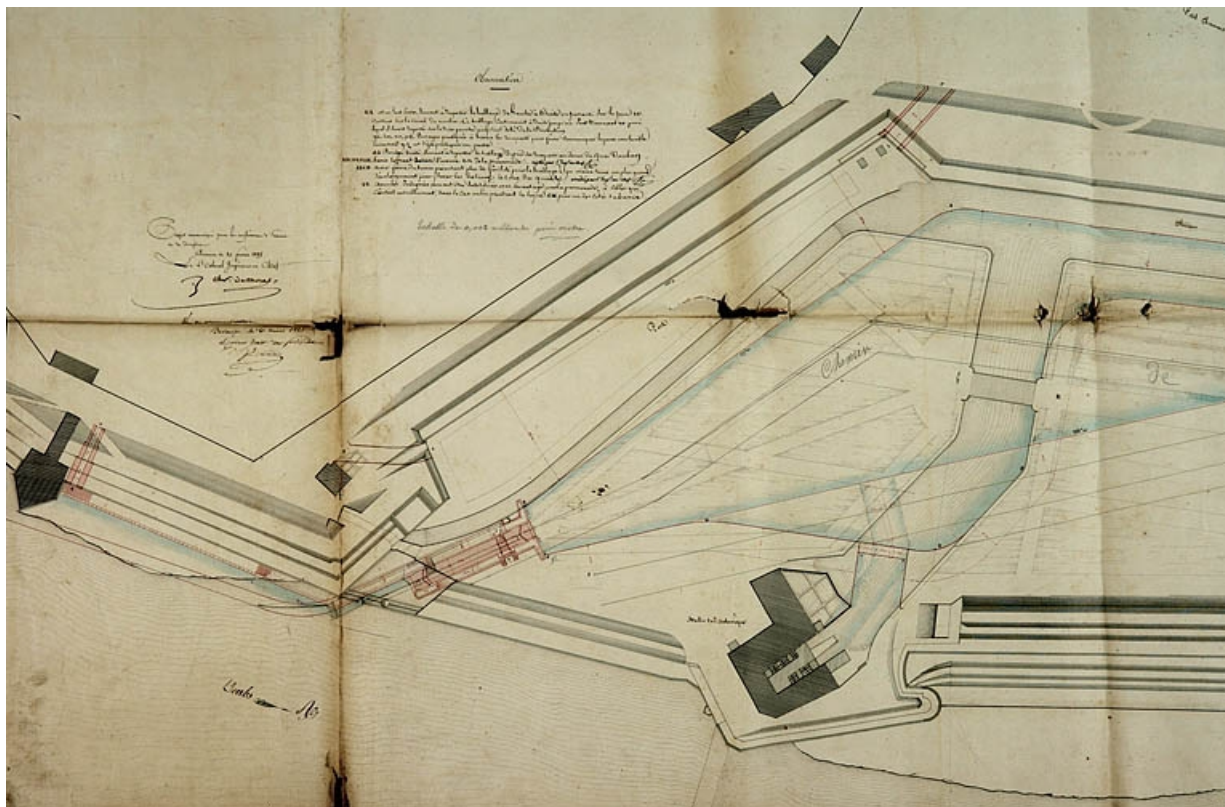
Plan général des ouvrages proposés dans la dérivation de Chamars [détail : partie amont], 1824. 25, Besançon
