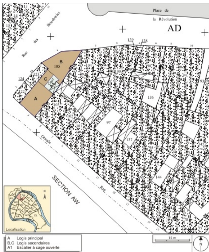
Plan masse et de situation. Extrait du plan cadastral, 1994, section AD. 25, Besançon Grande Rue 3, lieudit : îlot Chevanney
