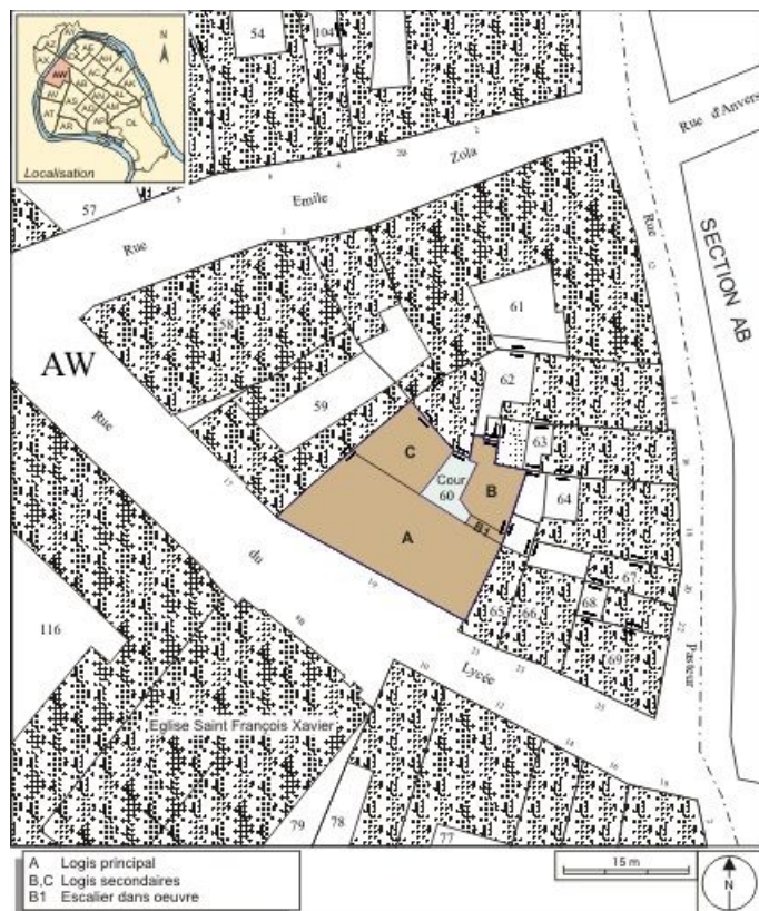
Plan masse et de situation. Extrait du plan cadastral, 1974, section AW. 25, Besançon, 19 rue du Lycée, lieudit : îlot d' Anvers
