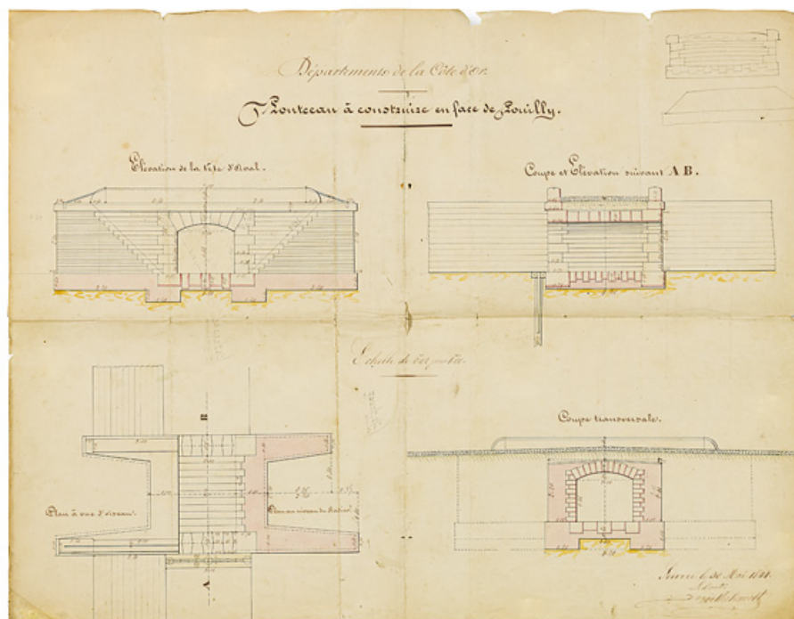
Ponceau à construire en face de Pouilly. Plan, coupe et élévation. Dessin, 30 mai 1844. 21, Seurre, lieudit : PK 190.5
