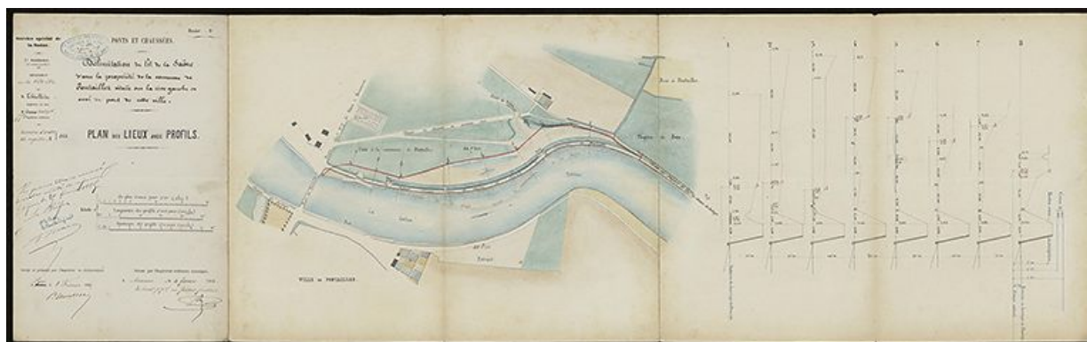
Délimitation du lit de la Saône d'avec la propriété de la commune de Pontailler située sur la rive gauche en aval du pont de cette ville. Plan des lieux avec profils. 1840.
