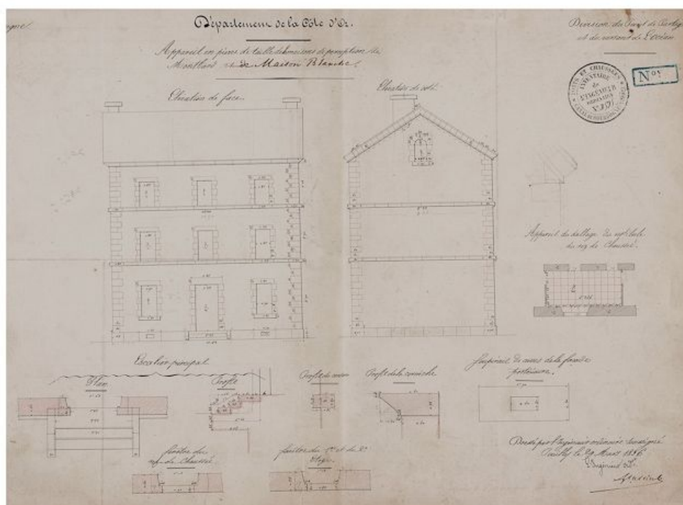
"Appareil en pierre de taille des maisons de perception de Montbard et de Maison-Blanche". Elévation de la façade et du pignon ; dallage ; soupirail ; éléments de l'escalier. 1836. (Archives départementales de la Côte-d'Or, Dijon)
