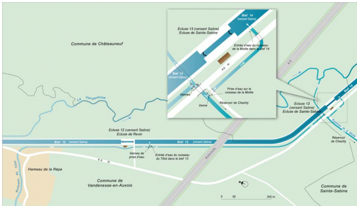
Plan schématique du réseau hydraulique des biefs 13 et 14 du versant Saône.
