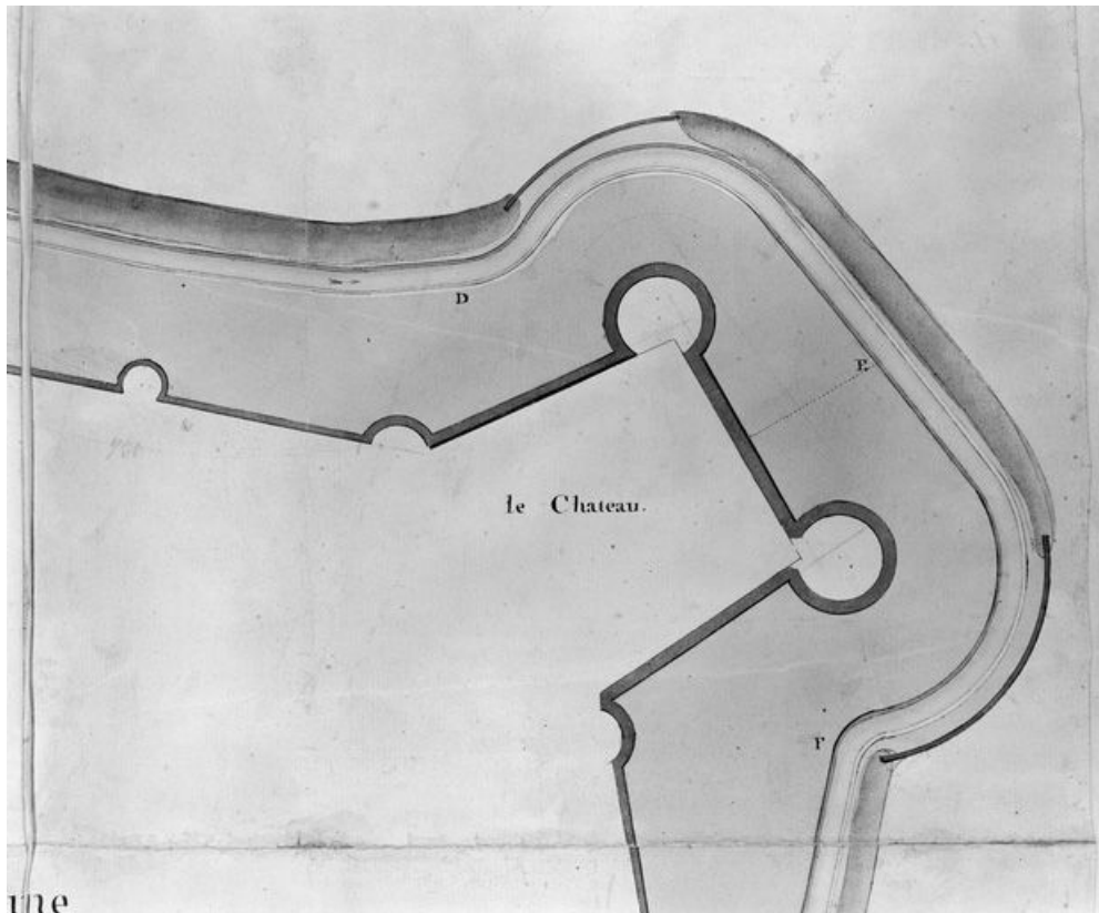
Plan de l'enceinte de Beaune levé en 1785 par François Pourcher, détail : le château. 21, Beaune rue du Château
