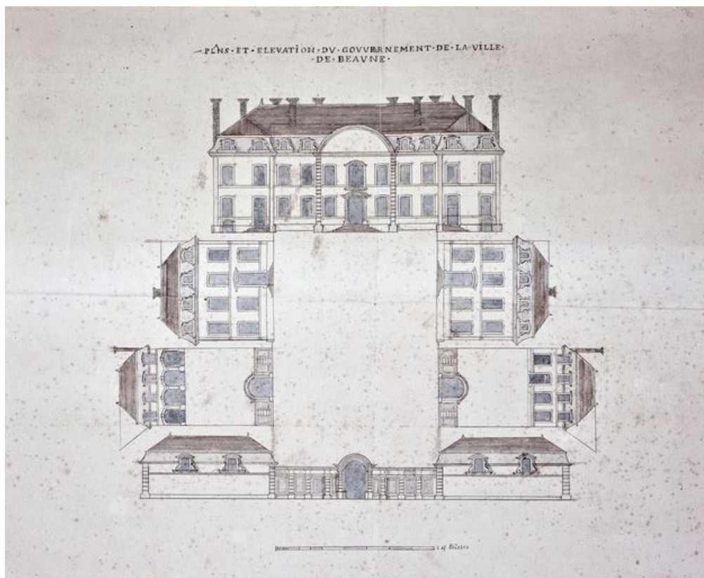
Projet [non réalisé] d'édifier un logement pour le gouverneur sur l'esplanade du château, signé Quinard, vers 1738. 21, Beaune rue du Château
