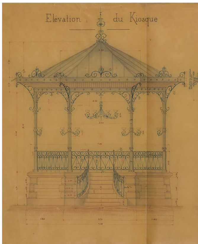
Ville de Châtillon-sur-Seine. Etablissement d'un kiosque à musique [... Détail : élévation]. 9 novembre 1908.
