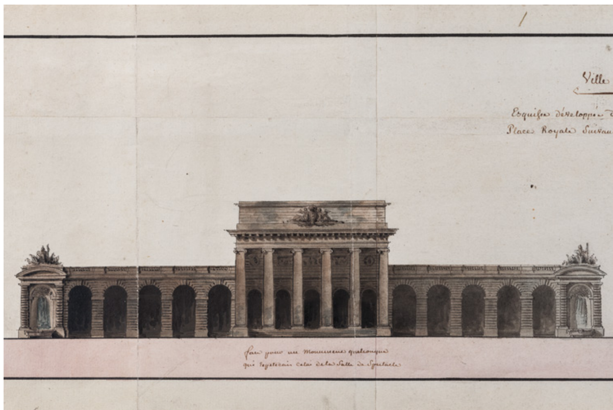
Ville de Dijon. Esquisse développée d'un projet de décoration de la Place royale [... 1er projet de salle de spectacle de Cellerier à l'emplacement du couvent des jacobines. Elévation du bâtiment symétrique]. S.d. [1785]. Légende : "Face pour un monument quelconque qui répéterait celui de la salle de spectacle".
