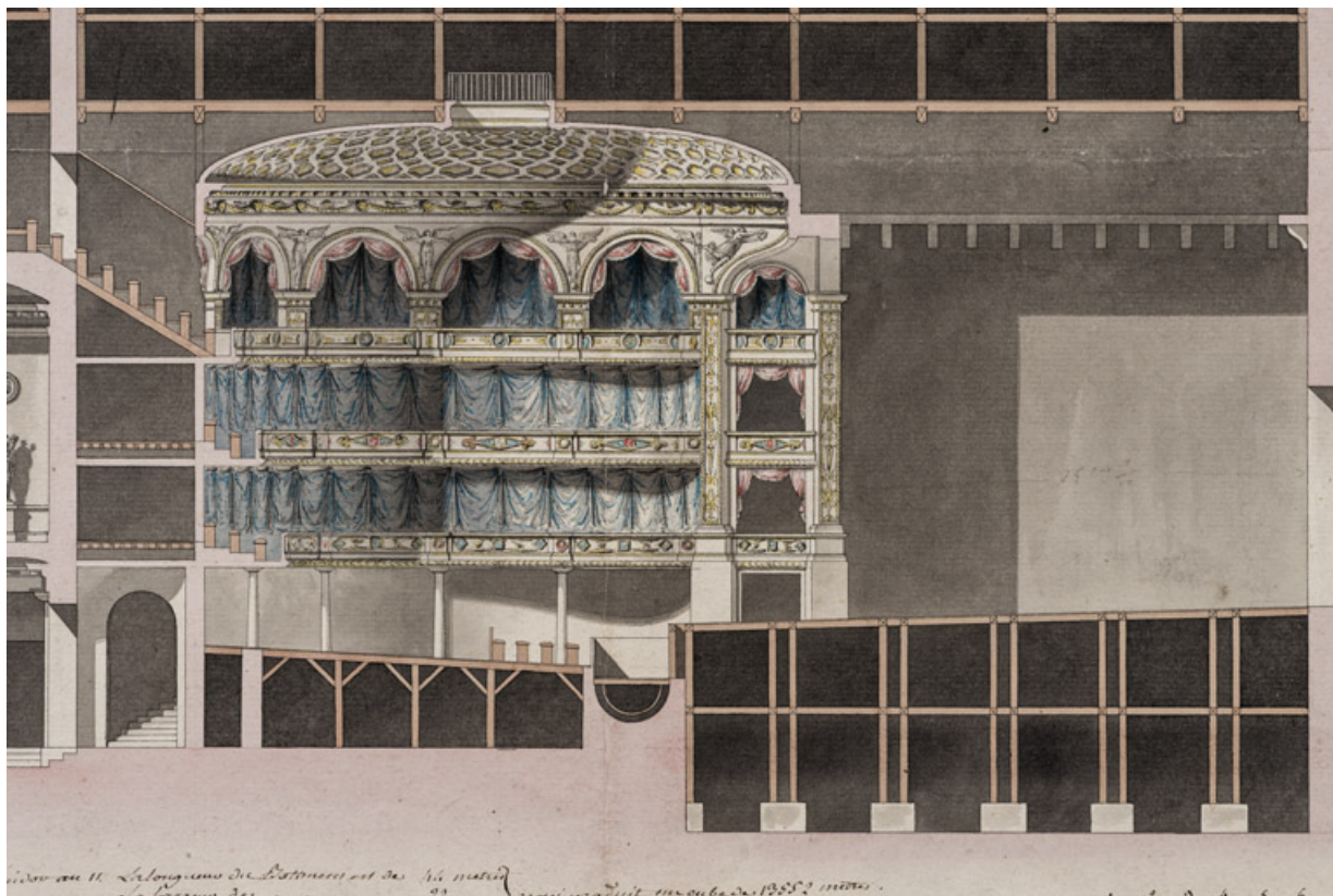
[Projet de salle de spectacle par Cellerier]. Ville de Dijon. Coupe sur le longueur de la salle de spectacle [détail]. S.d. [1803 ?]. 21, Dijon place du Théâtre
