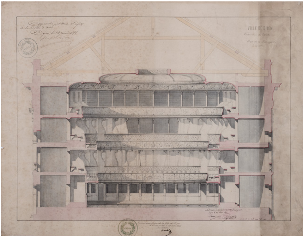
Ville de Dijon. Restauration du théâtre. Coupe de la face opposée à la scène. 28 mai 1855. 21, Dijon place du Théâtre
