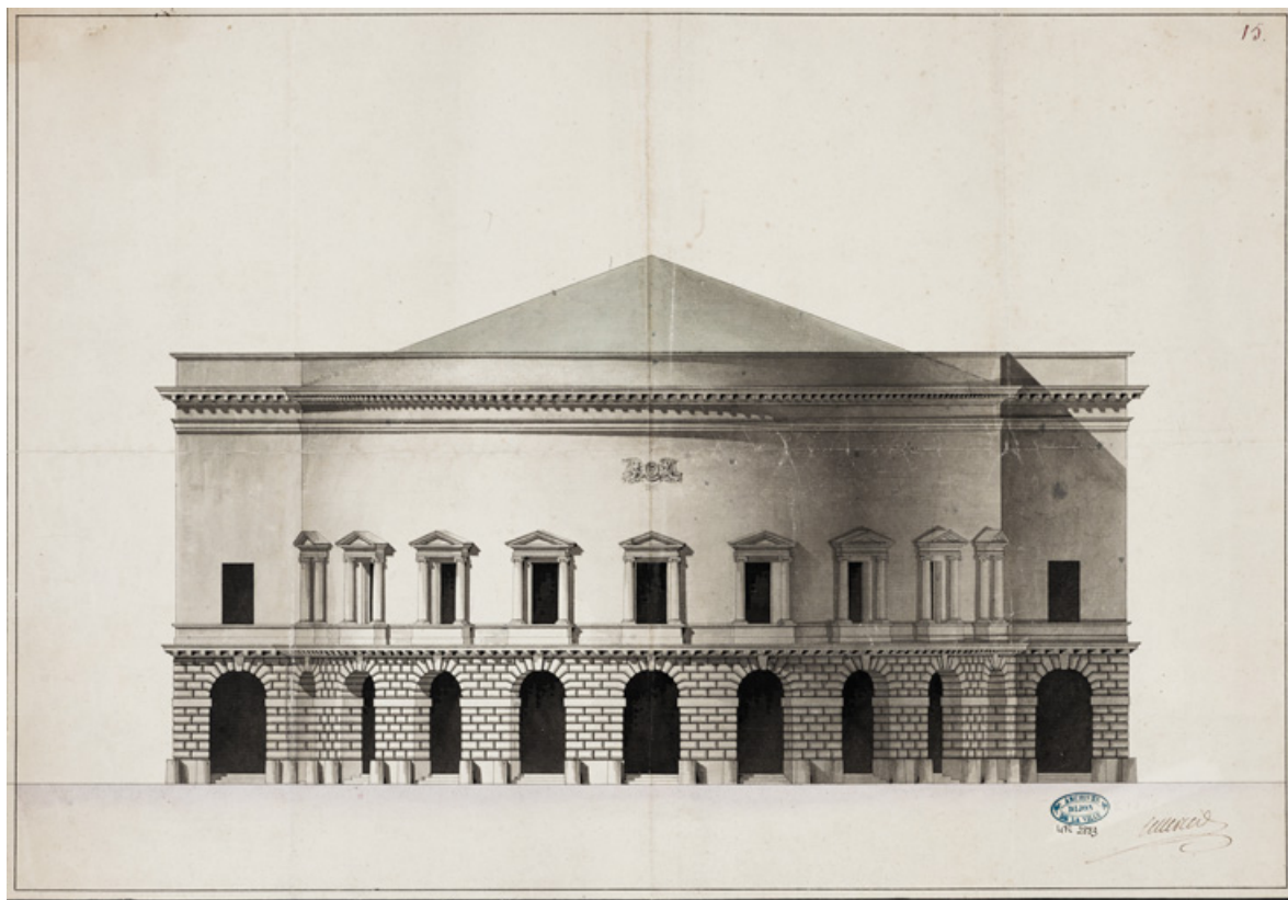
[3e projet de salle de spectacle de Cellier en 1787 à l'emplacement du couvent des jacobines : élévation]. 5 décembre 1787. 21, Dijon place du Théâtre
