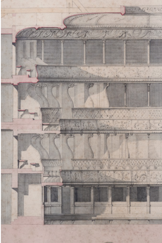
Ville de Dijon. Restauration du théâtre. Coupe de la face opposée à la scène [détail]. 28 mai 1855. 21, Dijon place du Théâtre
