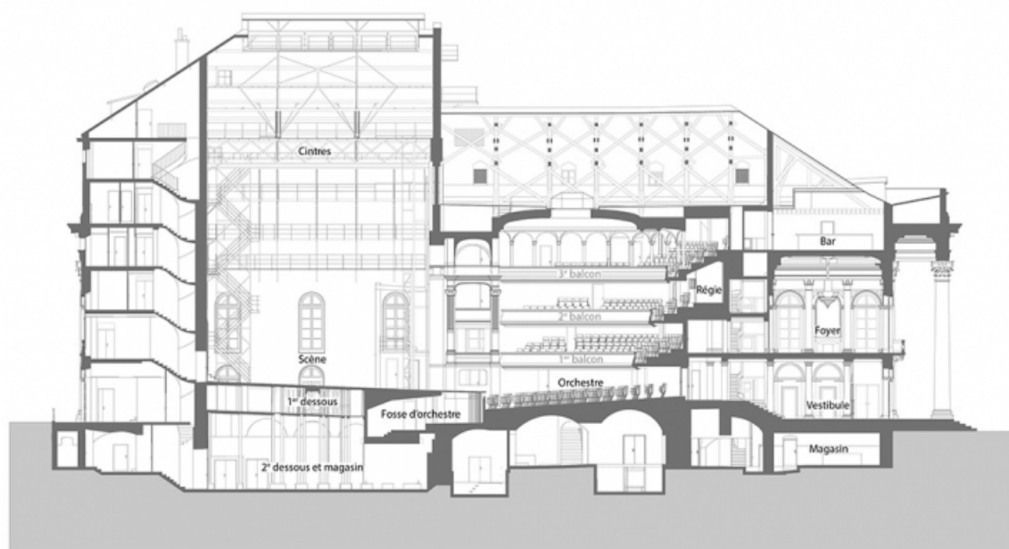
Coupe longitudinale. D'après une coupe non datée fournie par le service des Données patrimoniales, direction Bâtiments et Energies de Dijon Métropole.
