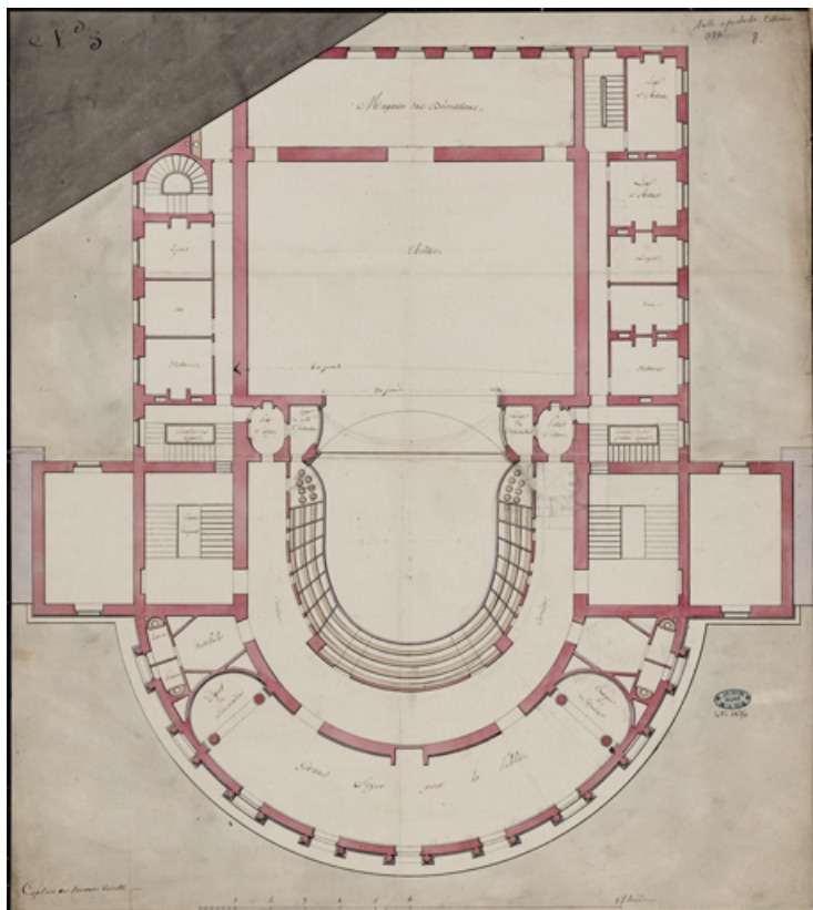
[3e projet de salle de spectacle de Cellerier à l'emplacement du couvent des jacobines : plan du 1er balcon]. 5 décembre 1787. 21, Dijon place du Théâtre
