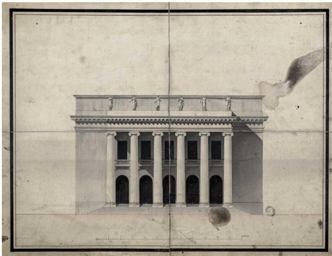
[2e projet de salle de spectacle à l'emplacement du couvent des jacobines, par Cellier : élévation]. S.d. [1786 ?]. 21, Dijon place du Théâtre
