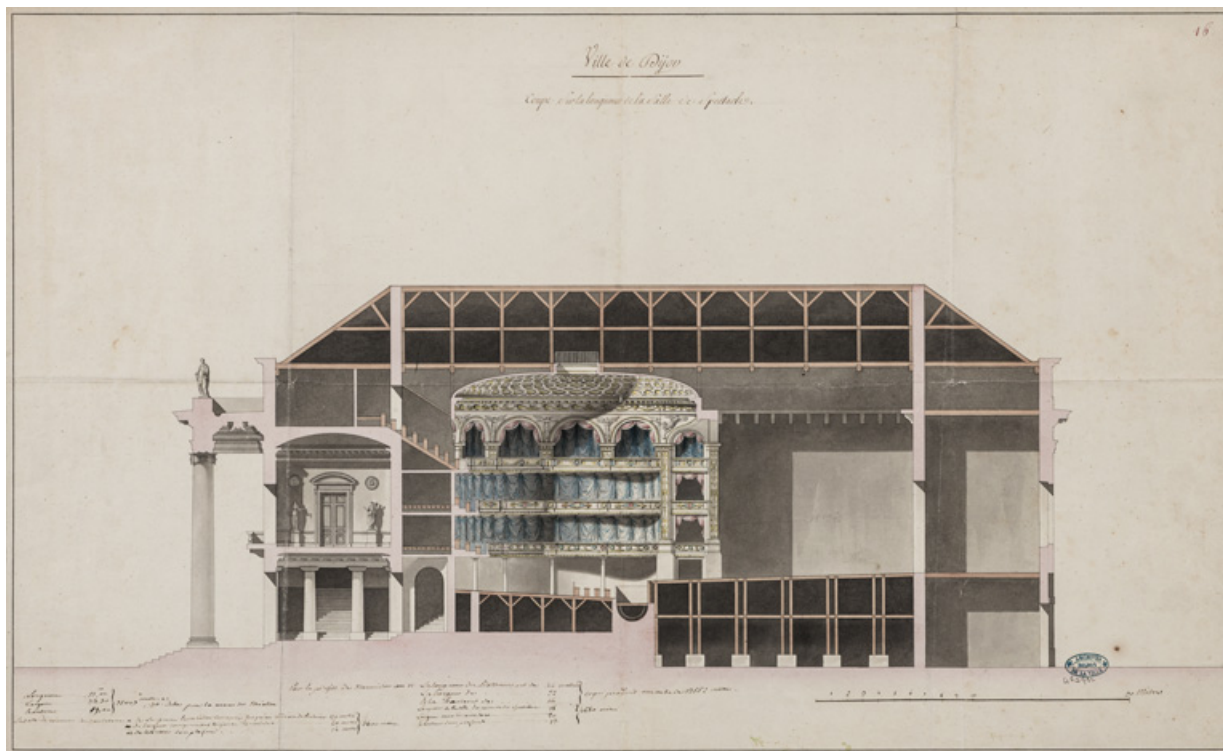
[Projet de salle de spectacle par Cellerier]. Ville de Dijon. Coupe sur le long de la salle de spectacle. S.d. [1803 ?]. 21, Dijon place du Théâtre
