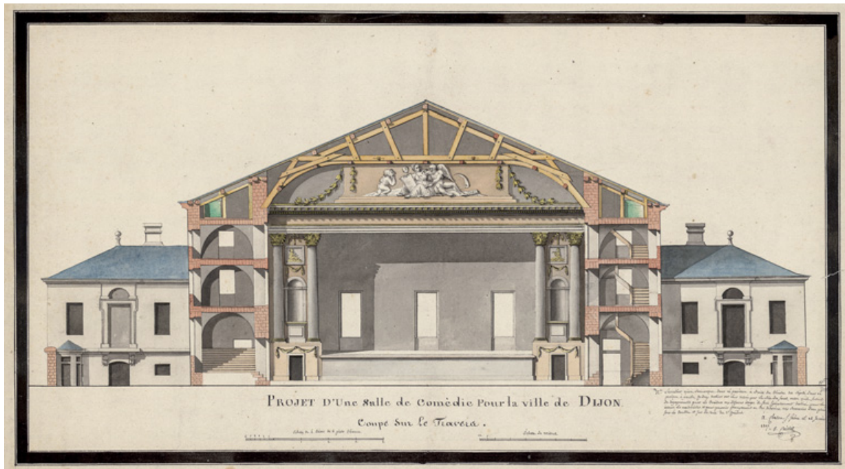
Projet d'une salle de Comédie pour la ville de Dijon. Coupe sur le travers [par E. Cailliet]. 12 janvier 1807. 21, Dijon place du Théâtre
