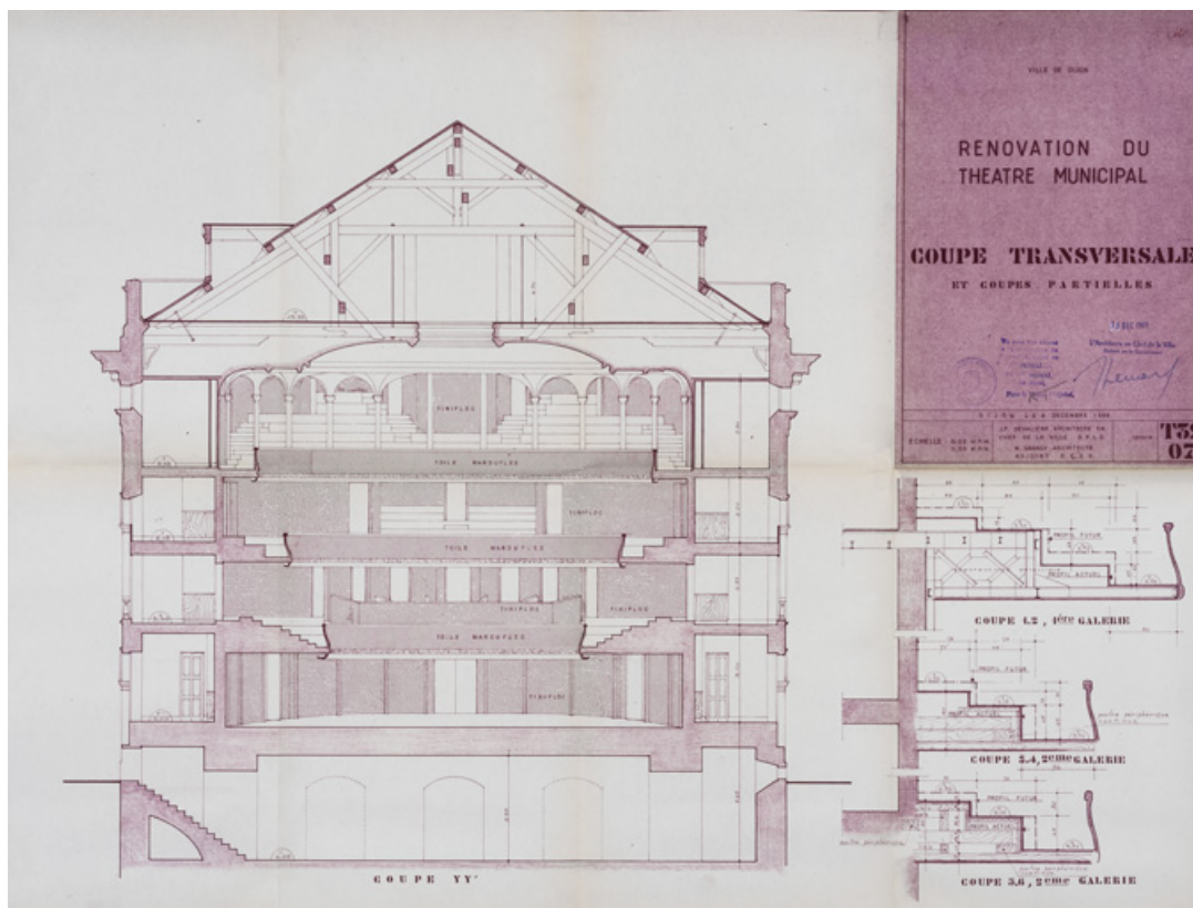
Rénovation du théâtre municipal. Coupe transversale et coupes partielles. T 32 07. 8 décembre 1969. 21, Dijon place du Théâtre
