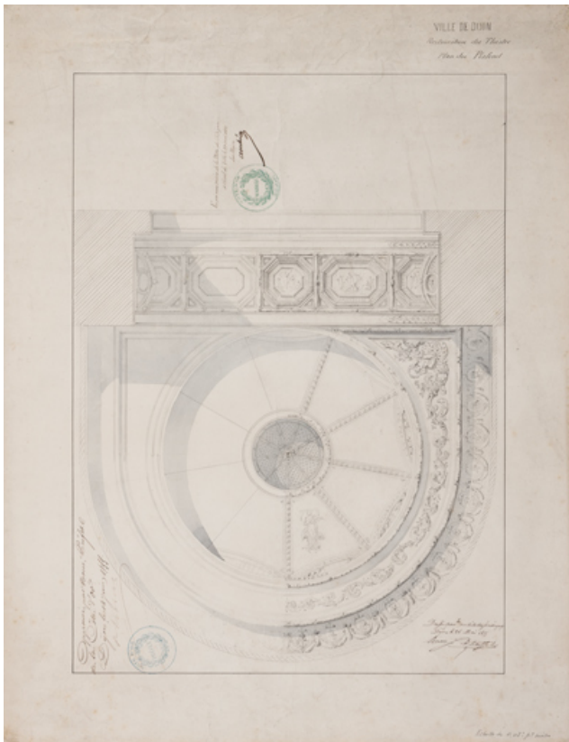
Ville de Dijon. Restauration du théâtre. Plan du plafond. 28 mai 1855. 21, Dijon place du Théâtre
