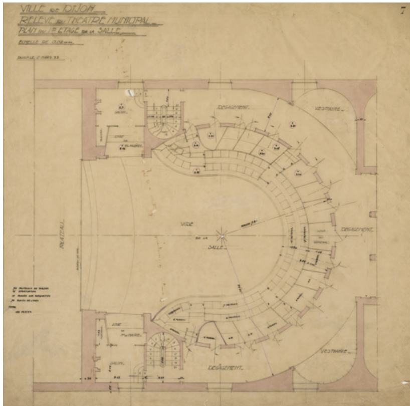
Ville de Dijon. Relevé du théâtre municipal. Plan du 1er étage de la salle. 17 mars 1933. 21, Dijon place du Théâtre
