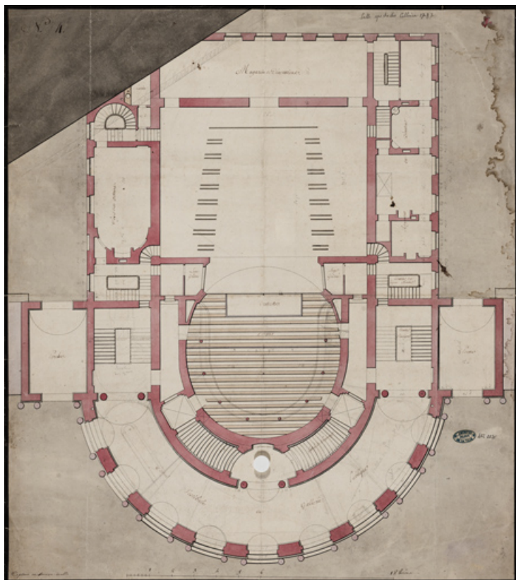
[3e projet de salle de spectacle de Cellerier à l'emplacement du couvent des jacobines : plan du rez-de-chaussée (variante)]. 5 décembre 1787.
