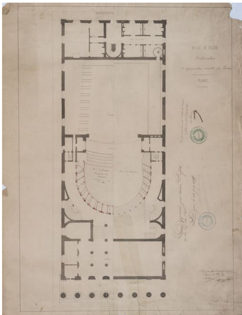
Ville de Dijon. Restauration et appropriation nouvelle du théâtre. Plans. 28 mai 1855. 21, Dijon place du Théâtre
