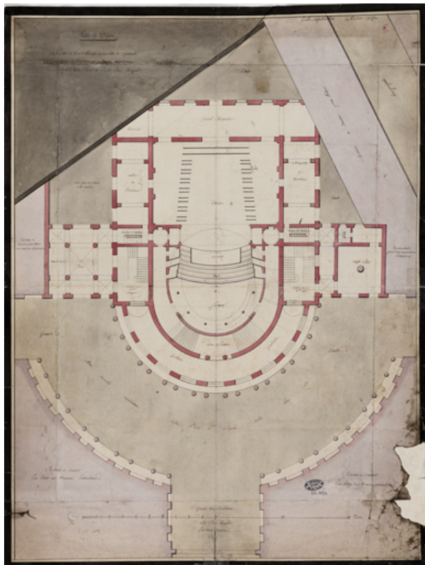
Plan du rez de chaussée de la salle de spetacle [sic] projetée sur l'emplacement du terrain appartenant à la ville [... Variante du 3e projet de Cellierier à l'emplacement du couvent des jacobines]. S.d. [1787].
