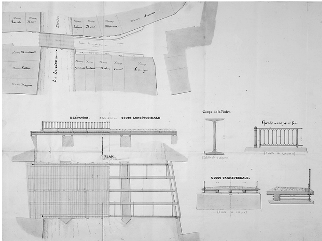
Projet de reconstruction en bois, 1872. 25, Montbéliard rue Saint-Hippolyte
