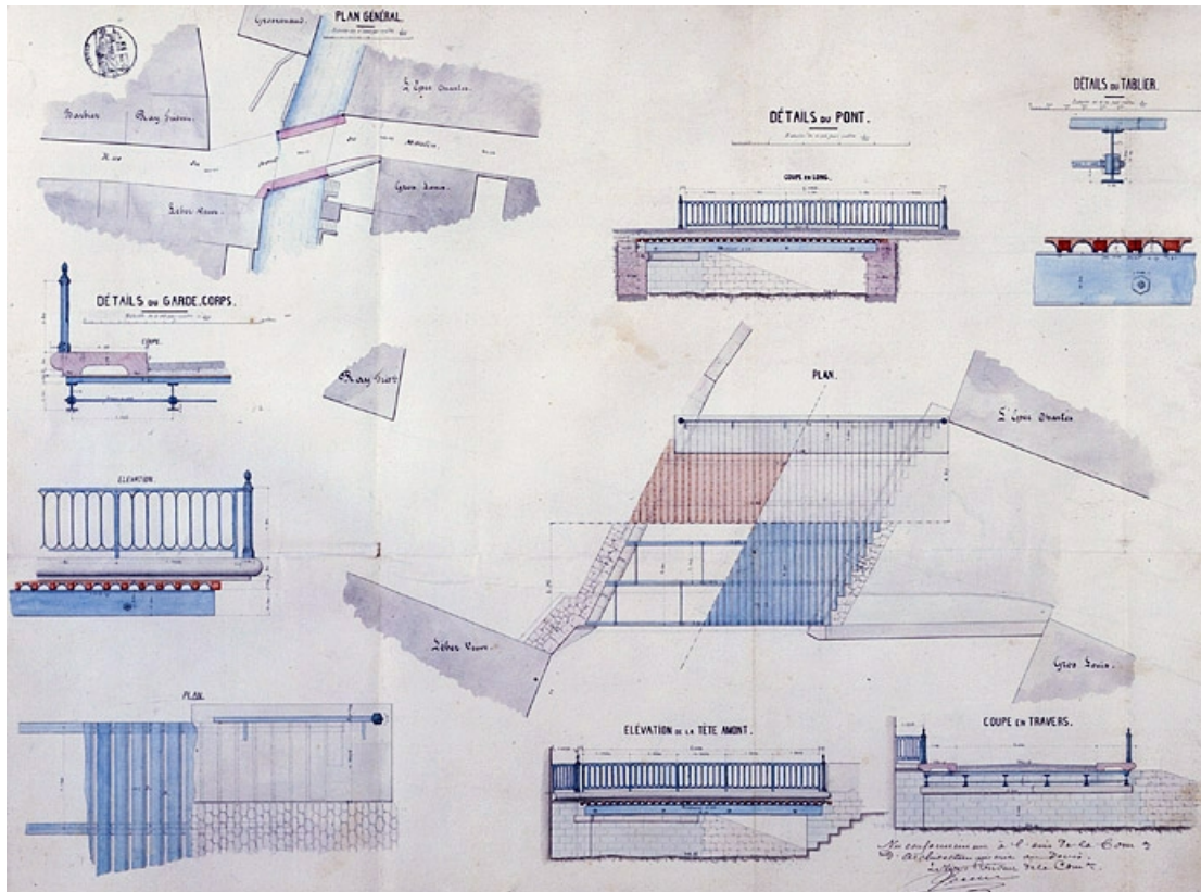
Projet de reconstruction en métal, 1873.
