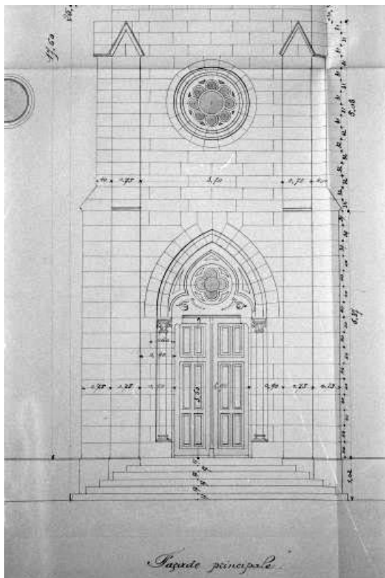
Projet de clocher : détail du portail.
