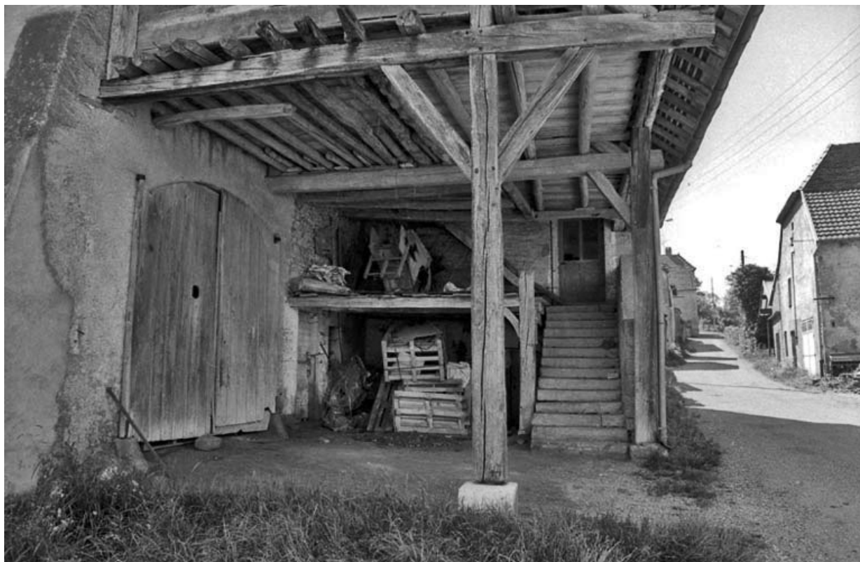
Détail : entrée de l'habitation sous auvent avec escalier extérieur en 1981.
