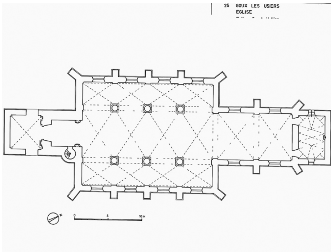
Plan au sol par J.-M. Demoly et Gilbert Poinso, 1975.
