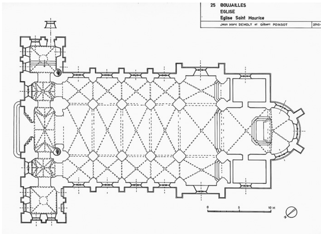
Plan au sol : relevé-croquis J.-M. Demoly et Gilbert Poinot, 1975.
