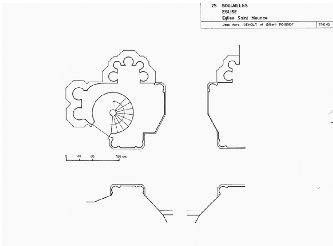
Plan des piliers d'entrée : relevé-croquis J.-M Demoly et Gilbert Poinot, 1975.
