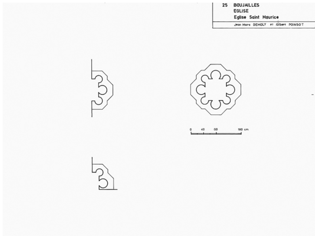
Plan des petits piliers : relevé-croquis J.-M Demoly et Gilbert Poinso, 1975.
