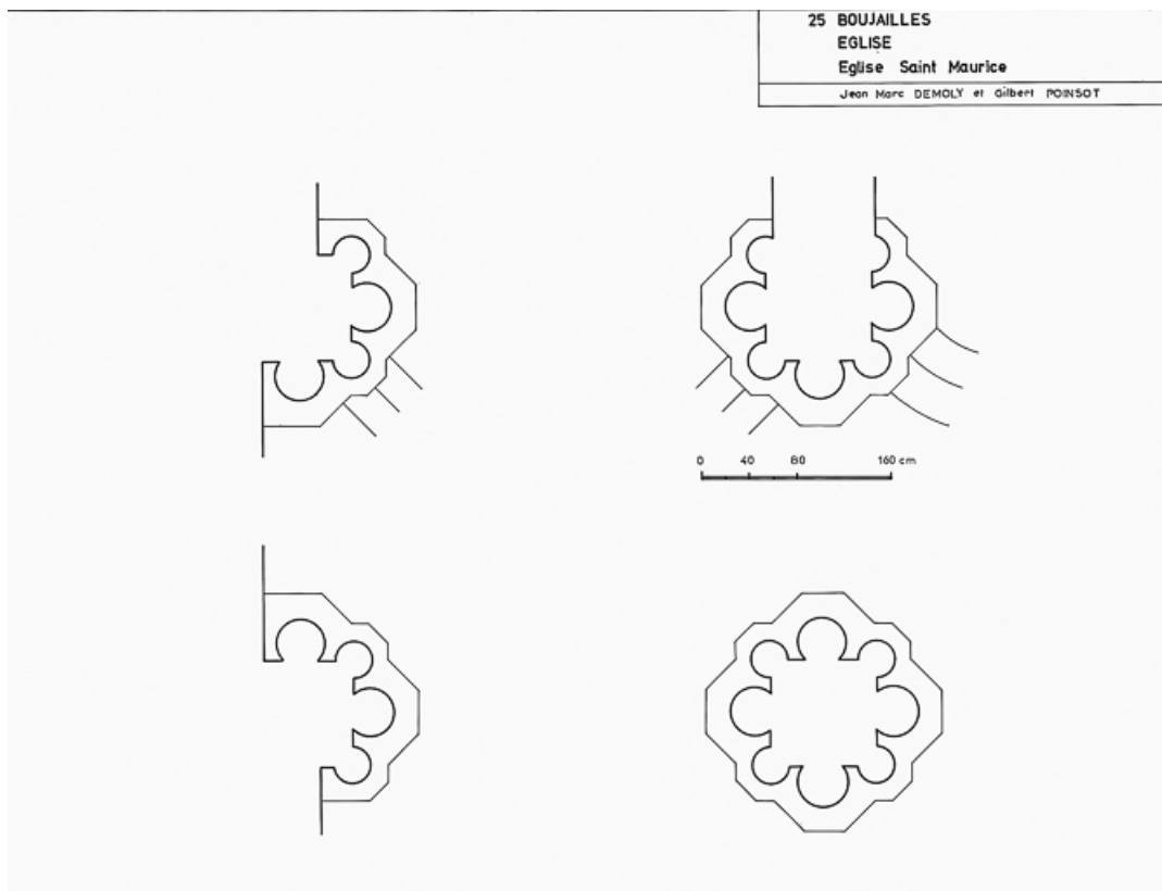
Plan des gros piliers : relevé-croquis J.-M Demoly et Gilbert Poinsoy, 1975.t, 1975. 25, Boujailles place de l' Eglise
