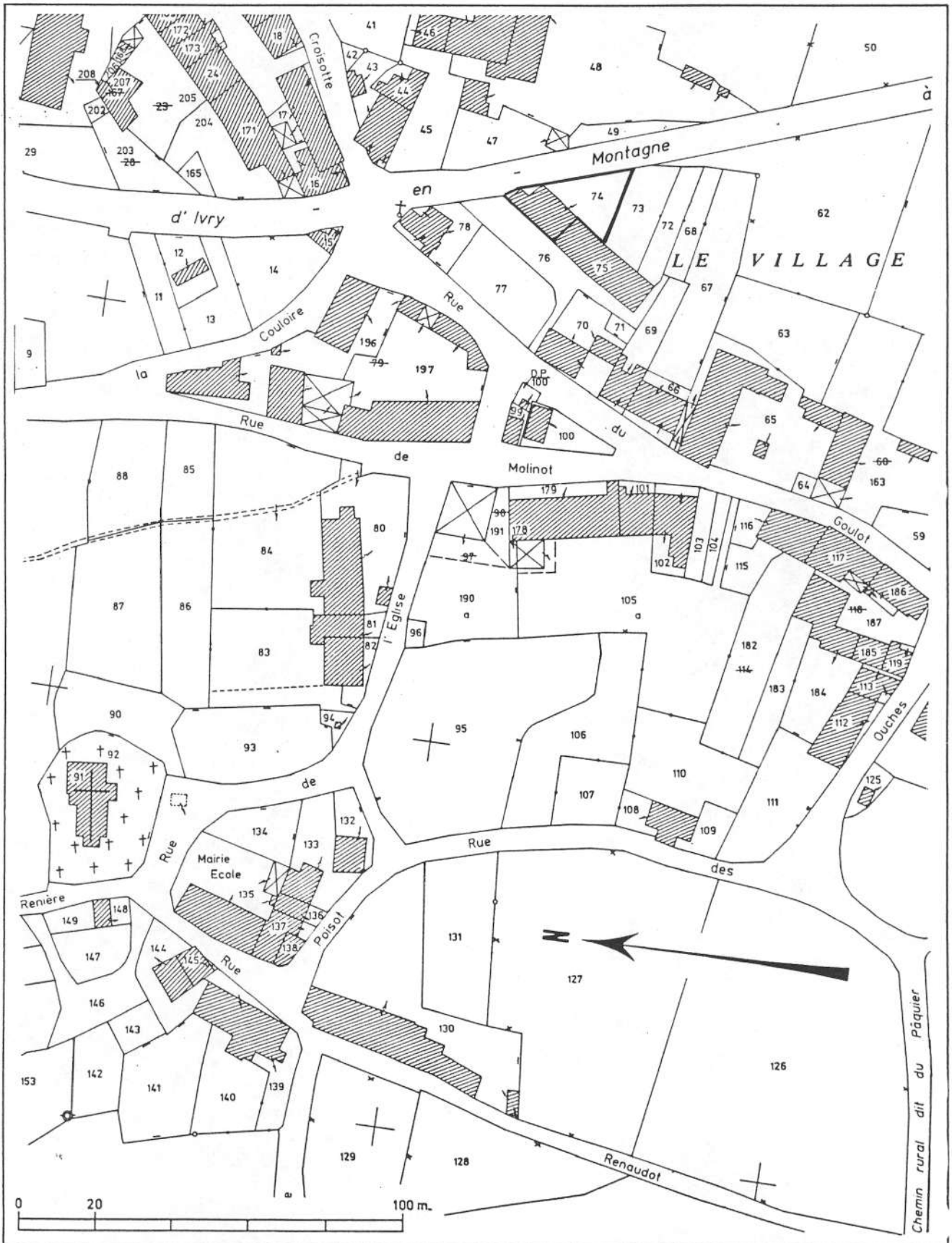
Pl. I - Plan de situation et plan-masse. Extrait du plan cadastral au 1:1000e, section AB de 1988.
