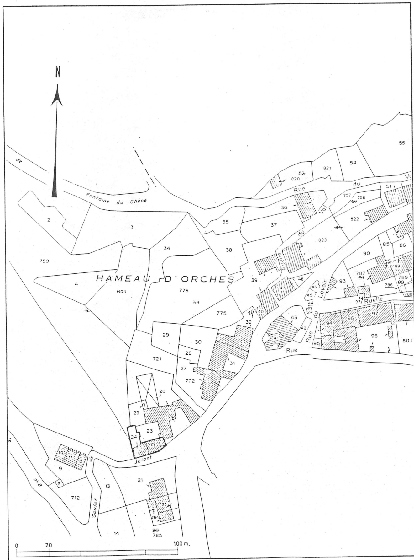
Pl. I - Plan de situation et plan-masse. Extrait du plan cadastral au 1:1000e, section B de 1984.
