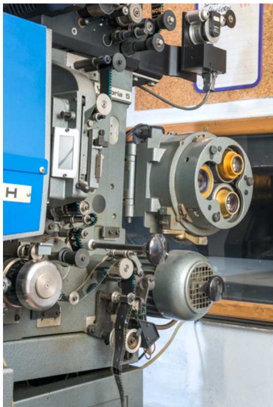
Chrono et tourelle porte-objectifs, de trois quarts. 71, Chauffailles, 50 rue Centrale
