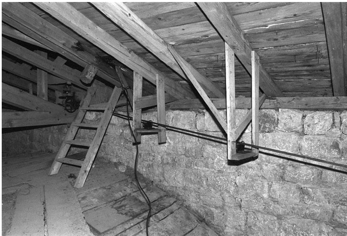
Tige de transmission du mouvement aux aiguilles du cadran extérieur sud.
