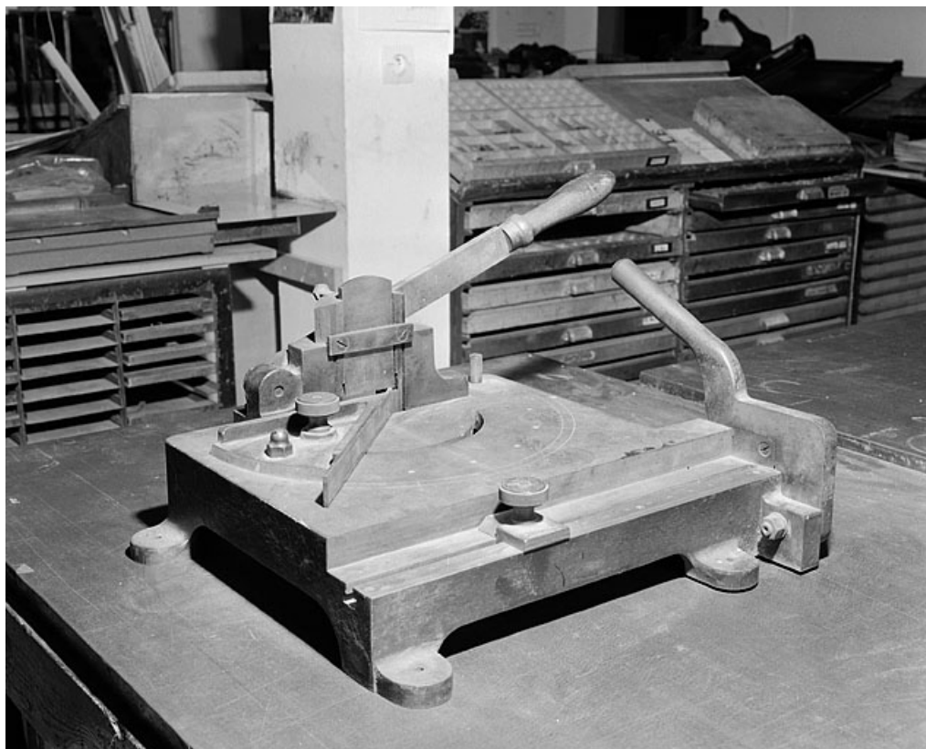
Vue d'ensemble d'un coupeur-biseauteur. "Couteau-rabot" pour les coupes obliques à gauche, "couteau-guillotine" pour les coupes de longueur à droite.
