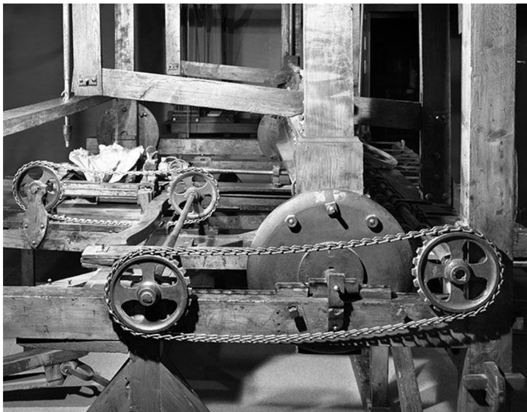
Face latérale droite. Aux premier et second plans, système de renvoi par chaîne permettant la rotation simultanée du modèle et des ébauchons.
