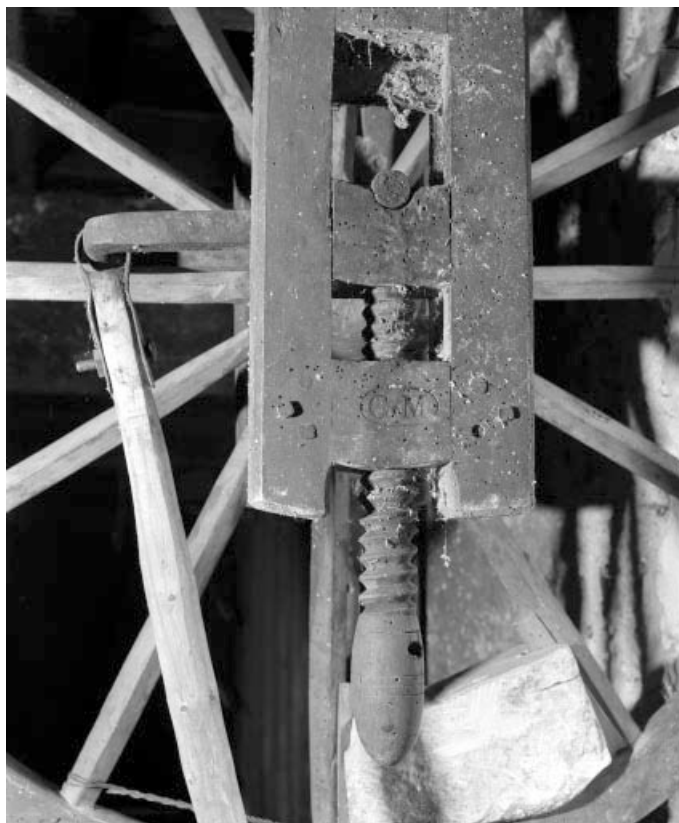
Vis de réglage en hauteur de l'axe de la roue et inscription. À l'arrière-plan, bielle, manivelle et poids équilibrant la roue.
