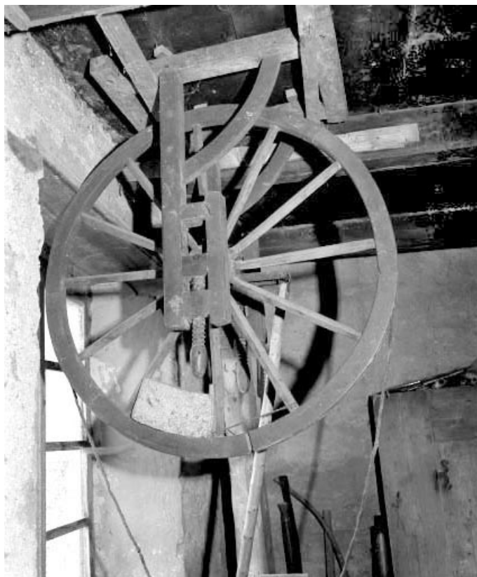
Roue motrice au plafond.
