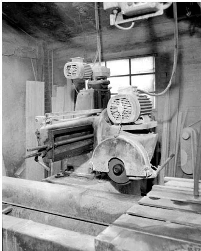
Débiteuse-moulineuse sud : bâti vertical, moteur et toupie.
