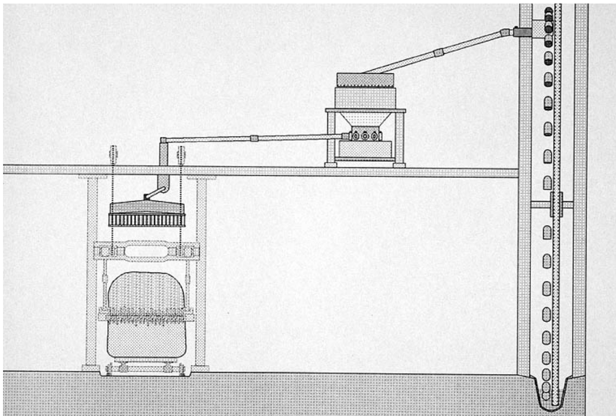
Schéma de fonctionnement de la norja et du système d'alimentation en " service " des châssis de scie.
