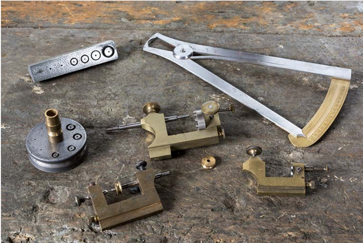
Exemple d'outils fabriqués dans l'atelier : outils à redresser les roues de cylindre (à gauche), au dixième (en haut à droite), à centrer et rapporter les pivots (les trois en bas autour d'un cuivrot, celui du haut étant dit à 12 cornets). 25, Les Gras
