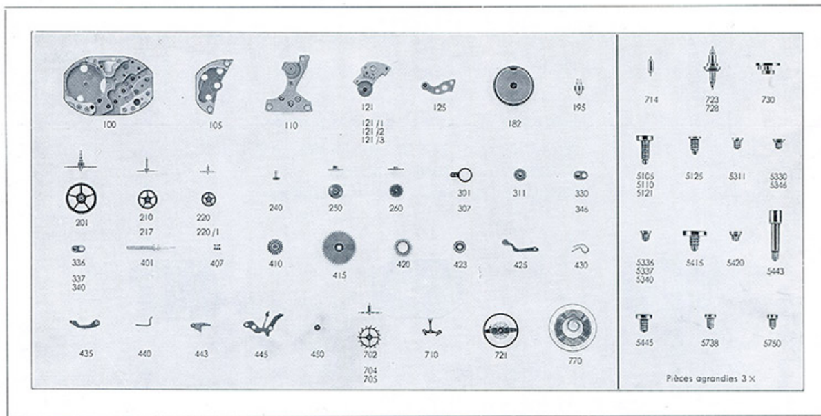
Calibre 5 1/4''' - 55 - 15 à 21 rubis [éclaté des fournitures], 1973. 25, Maîche
