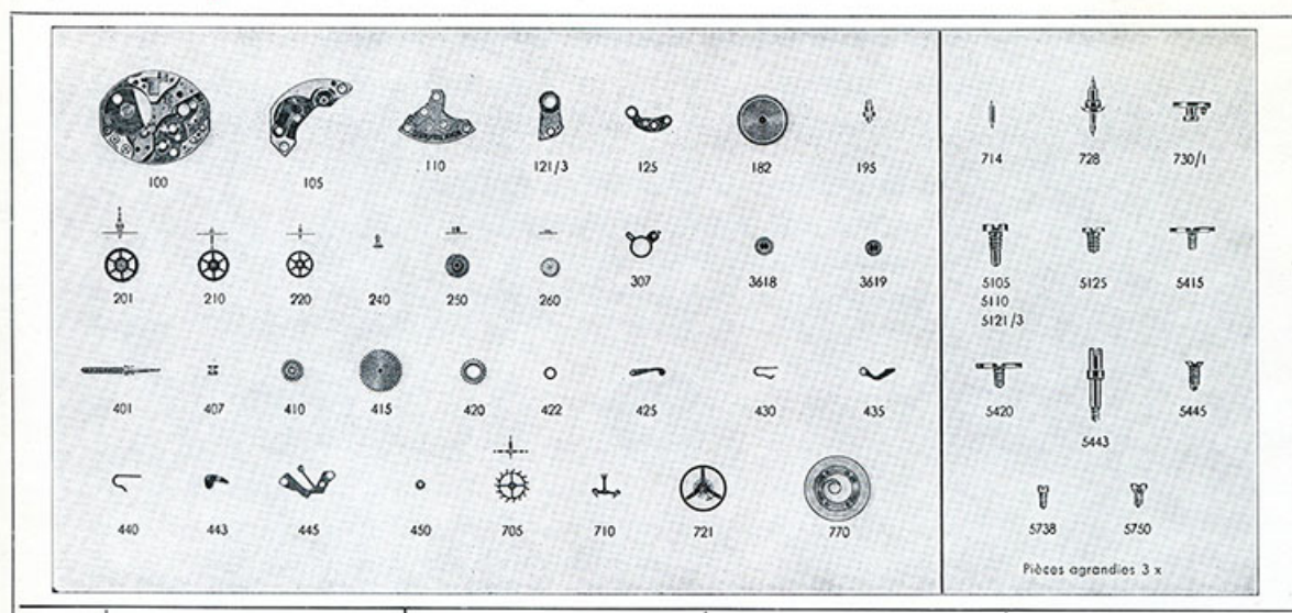
Calibre 5 1/2''' 68 - 17 rubis [éclaté des fournitures], 1973.
