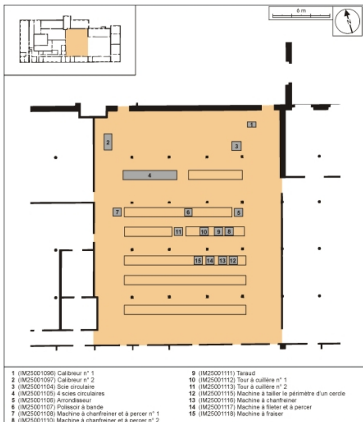
Plan de localisation des machines de la ligne de fabrication des têtes de pipe en merisier. 25, Baume-les-Dames rue des Pipes, lieudit : Gondé
