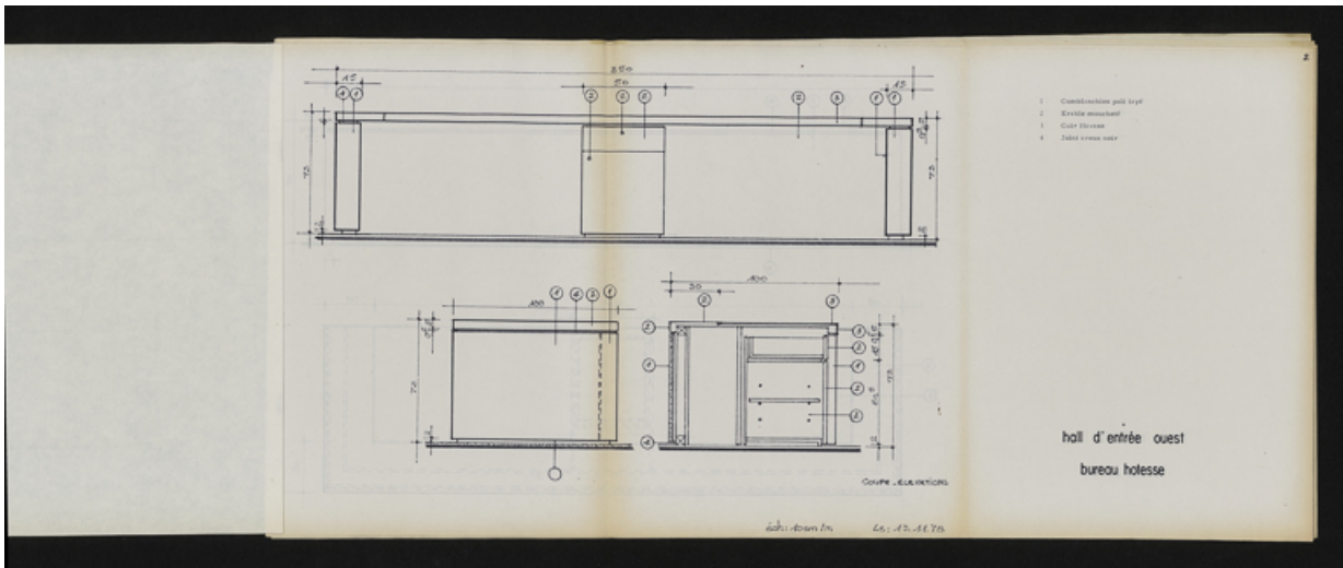
Carnet de détails et principes - hall d'entrée ouest : bureau des hôtesse, coupe et élévations, 13 novembre 1978. Boyer, Michel (architecte d'intérieur) (Archives départementales de la Côte-d'Or, Dijon, 32 J 106)
