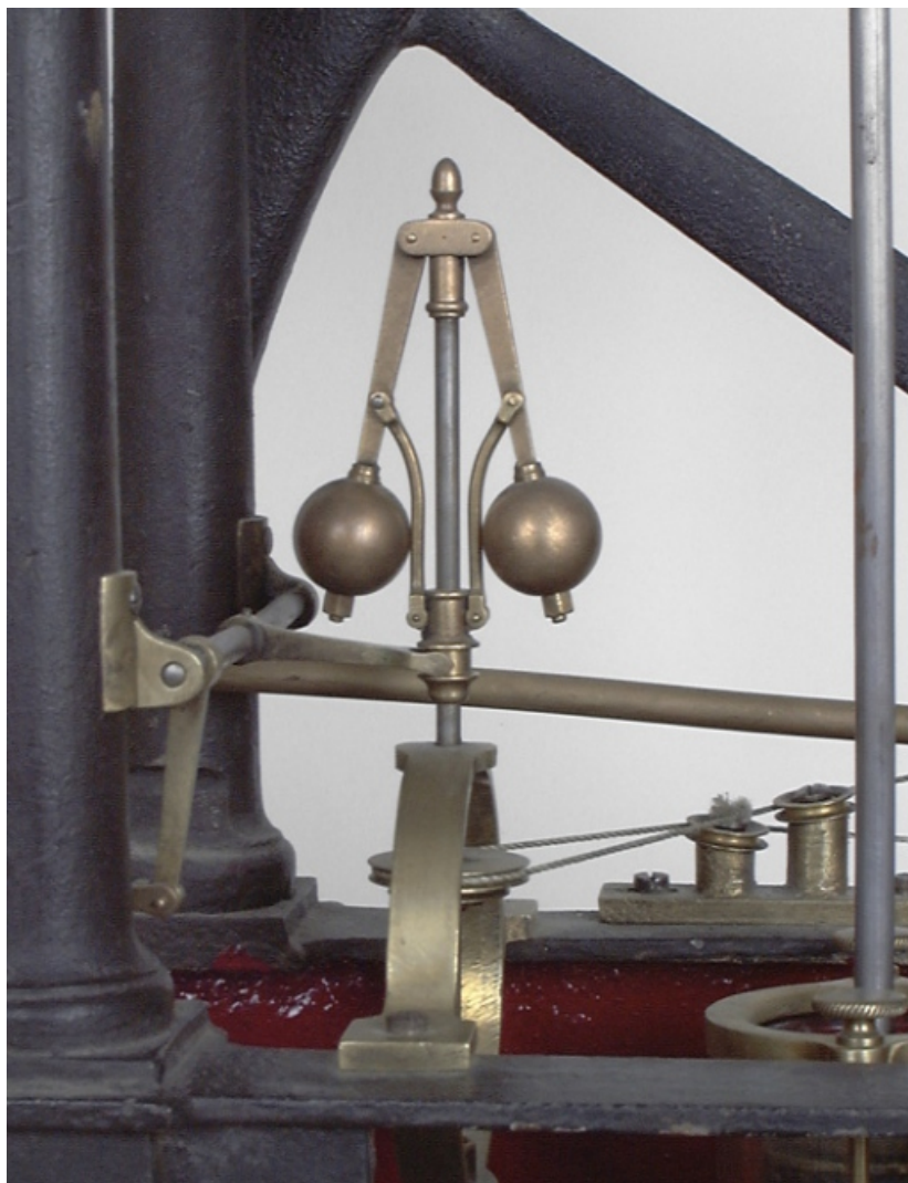
Détail du régulateur à boule. 21, Dijon, 16 boulevard Thiers
