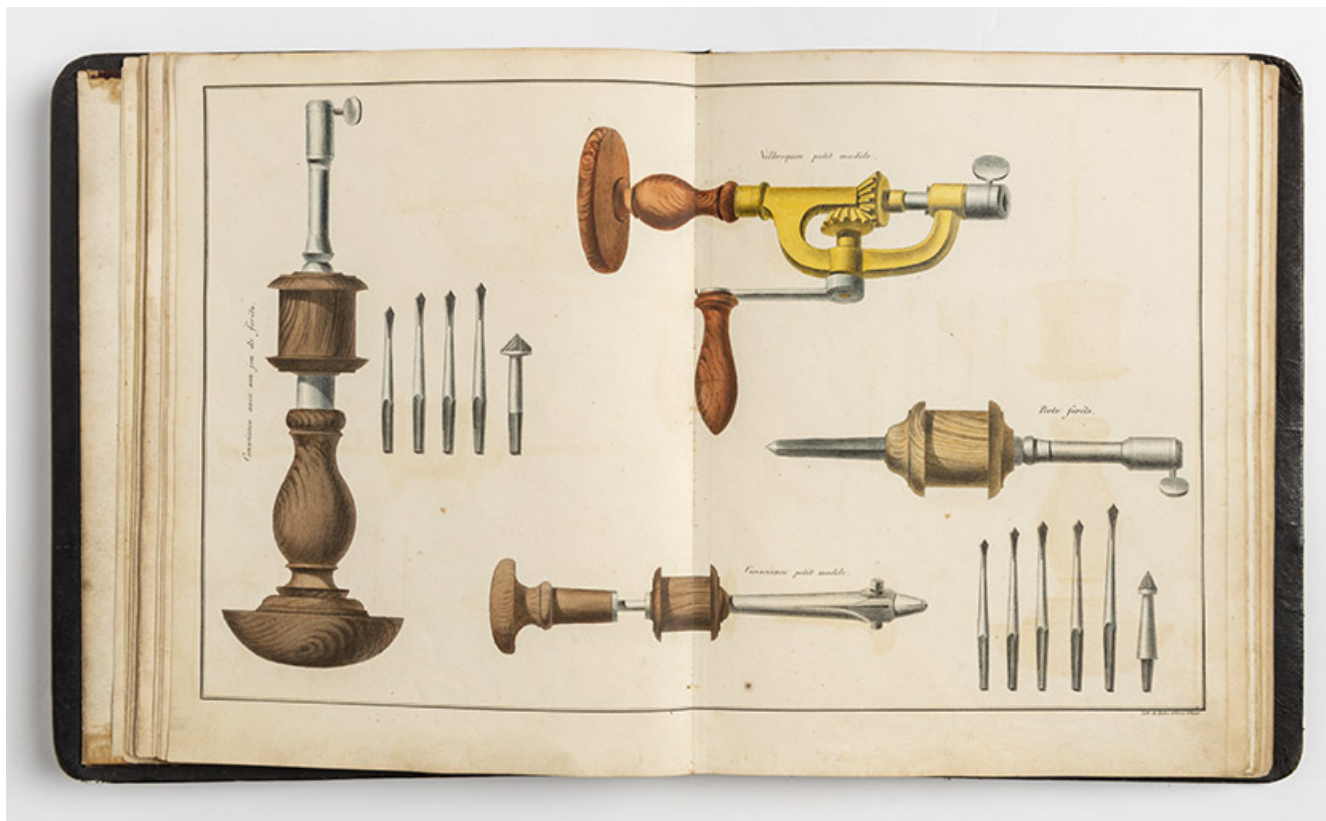
[Outillage : vilebrequin, "conscience", porte-forets : planche de catalogue], 1835.
