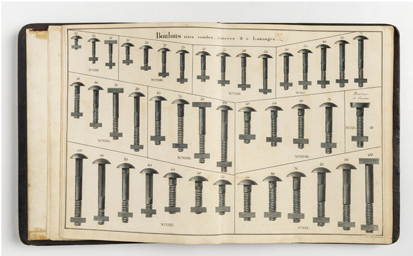
Boulons têtes rondes, carrées & à losanges [planche de catalogue], 1835. 90, Beaucourt
