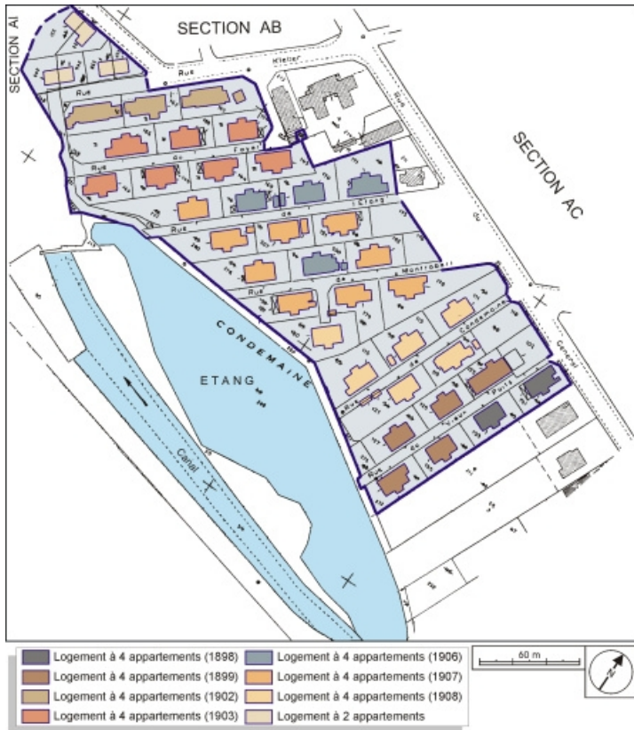
Plan-masse et de situation. Montage d'extraits de plan cadastral, 1984, sections AH et AI, 1:1000, le tout réduit à 1:2000. 90, Grandvillars, lieudit : cité Condemaine
