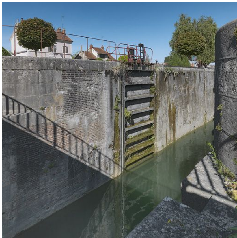
Site d'écluse vu d'amont : bajoyer en brique.
