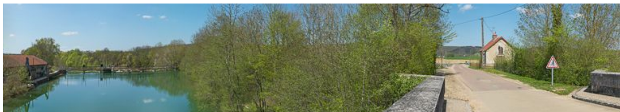
Vue panoramique d'un pont sur l'Armançon : de gauche à droite, l'Armançon avec un barrage, la maison éclusière. 89, Tanlay, lieudit : bief 91 du versant Yonne
