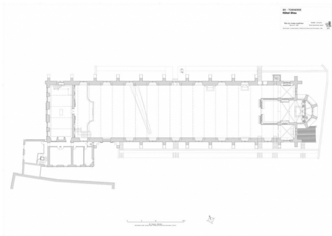
plan régulier du rez-de-chaussée, niveau supérieur
