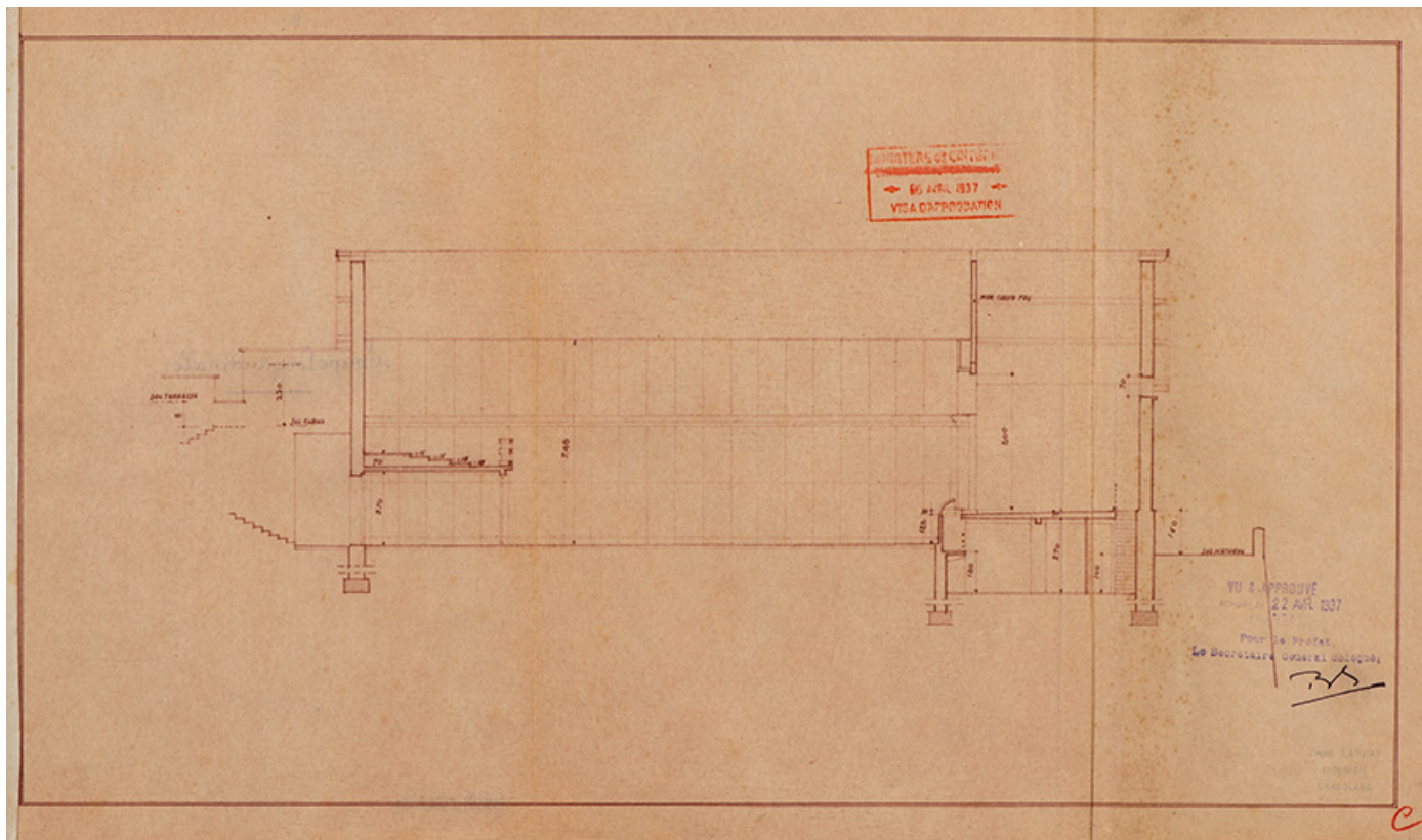
Ville de Charolles. Foyer municipal. Coupe longitudinale. S.d. [Visa du 16 avril 1937]. 71, Charolles, 40B rue Baudinot
