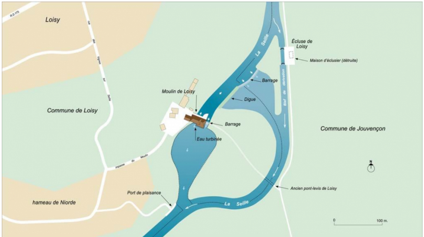
Plan schématique du site de l'écluse de Loisy, des barrages, du pont et du moulin de Loisy. 71, Loisy
