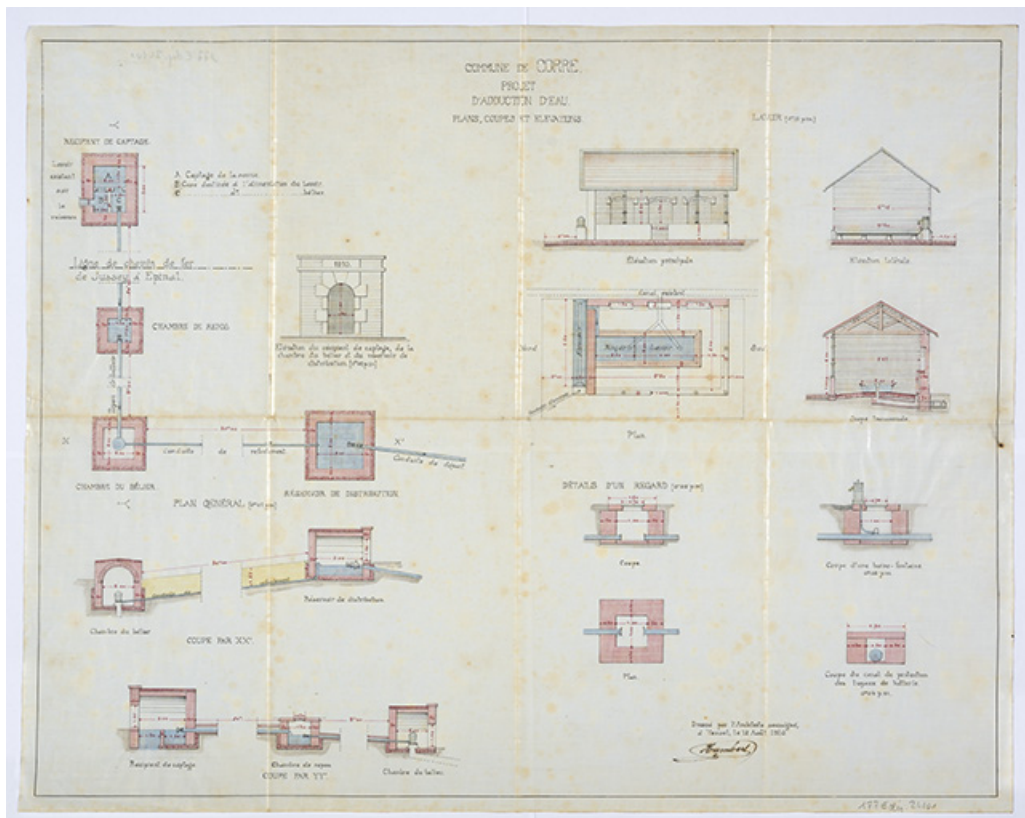
Commune de Corre. Projet d'adduction d'eau. [plans, coupes, élévations.] 1910 70, Corre
