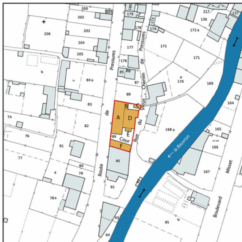
Plan-masse et de situation. Source : Direction générale des Finances Publiques - Cadastre ; mise à jour 2023, section CC, 1/1 000. 58, Clamecy, 41 route de Pressures
