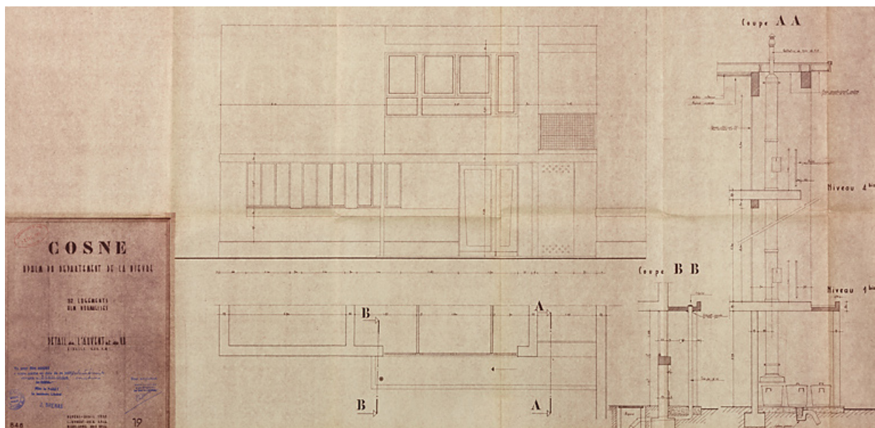
Opération de 32 logements, plan et élévations de détail de l'avant et du vide-ordure, L. Robert et M. Guillaume, avril 1955. (Archives municipales Cosne-Cours-sur-Loire, 200 W 16 - PC 722)
