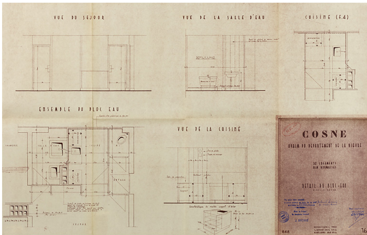
Opération de 32 logements, plans et élévations de détails du bloc-eau, L. Robert et M. Guillaume, avril 1955. (Archives municipales Cosne-Cours-sur-Loire, 200 W 16 - PC 722)
