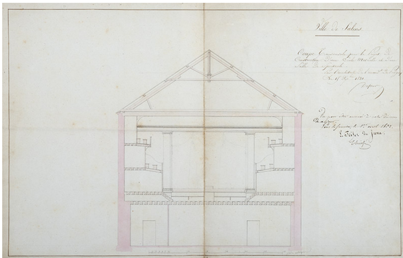
Coupe transversale pour le projet de construction d'une école mutuelle et d'une salle de spectacle, 1831. 39, Salins-les-Bains rue de la République
