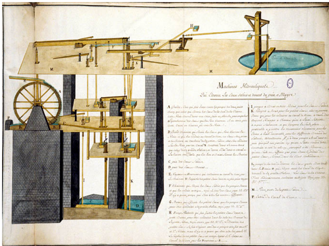
Machines Hydrauliques Qui Elèvent Les Eaux salées et douces du puits à Muire.
