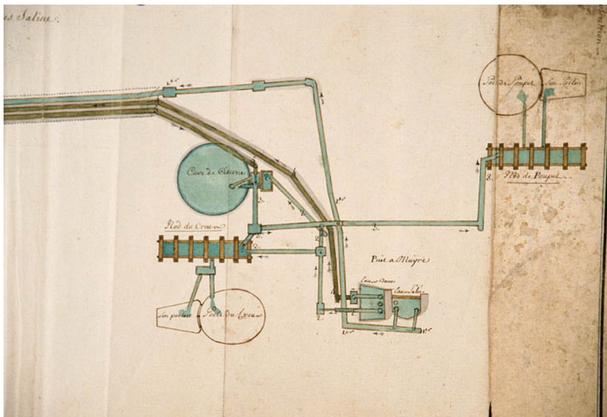
Plan des Différents Cours des Eaux salées et douces [... : détail du puits à muire et des bernés du Creux et du Poupet]. 39, Salins-les-Bains, 2 place des Alliés et de la Résistance
