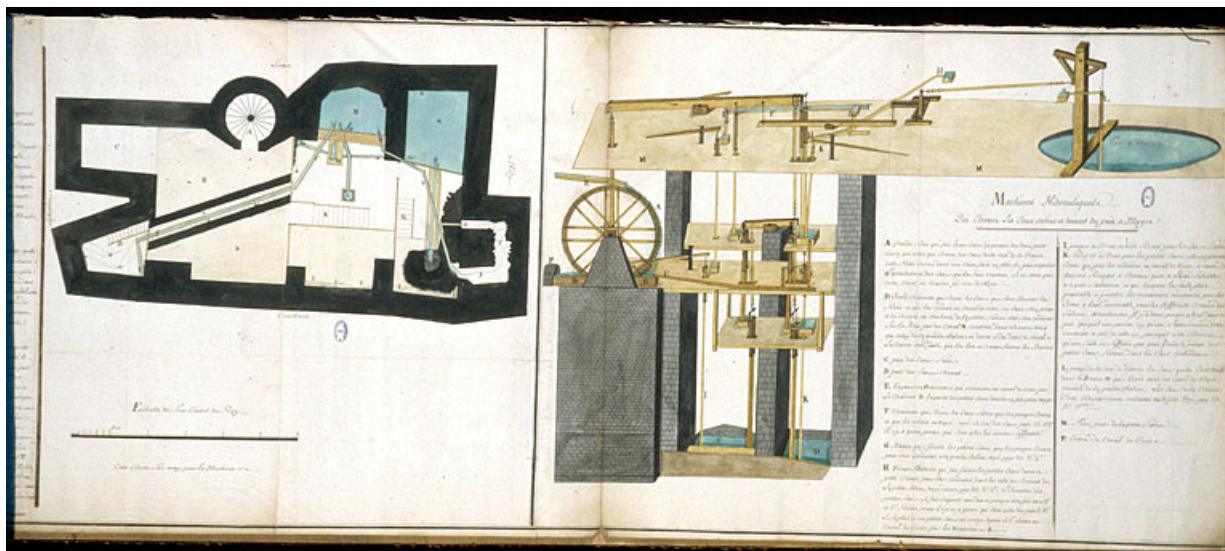
Plan des Sources du puit a Muire, a la petite Saline [et] Machines Hidrauliques Qui Elèvent Les Eaux salées et douces du puit à Muire.
