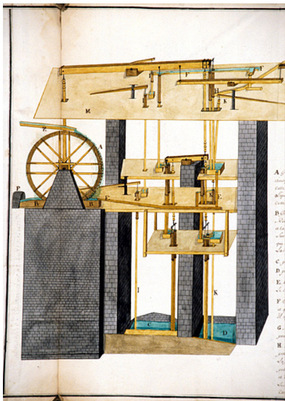
Machines Hydrauliques Qui Elèvent Les Eaux salées et douces du puit à Muïre [partie gauche du dessin].
