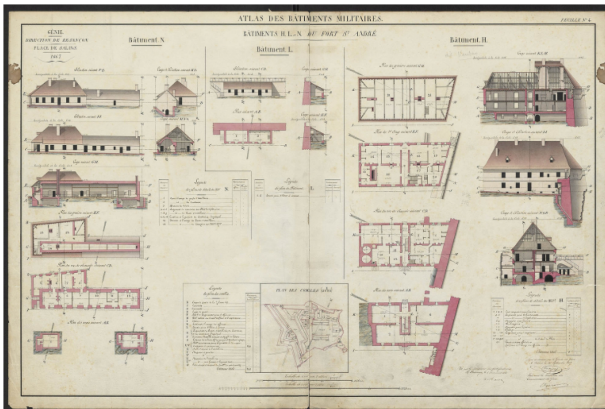
Atlas des bâtiments militaires. Génie. Direction de Besançon. Place de Salins. Bâtiments H, L et N du Fort St-André. 1867. 39, Salins-les-Bains chemin communal du Fort Saint-André, lieu dit : Fort Saint-André
