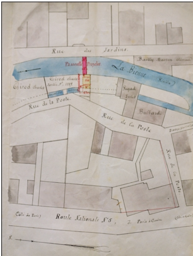
Construction d'une passerelle en fer sur la rivière de Bienne [...], 1896. 39, Morez quai Aimé Lamy
