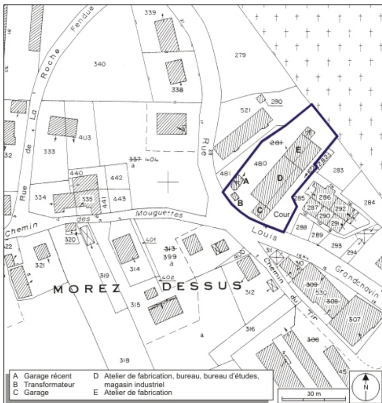
Plan-masse et de situation. Extrait du plan cadastral, 1980, section A1, échelle 1:1000. 39, Morez, 18 rue Louis Grandchavin
