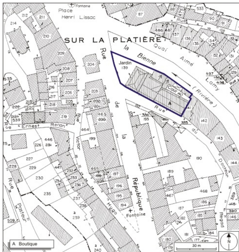
Plan-masse et de situation. Extrait du plan cadastral, 1980, section A1, échelle 1:1000. 39, Morez, 1-3 rue du Docteur Regad
