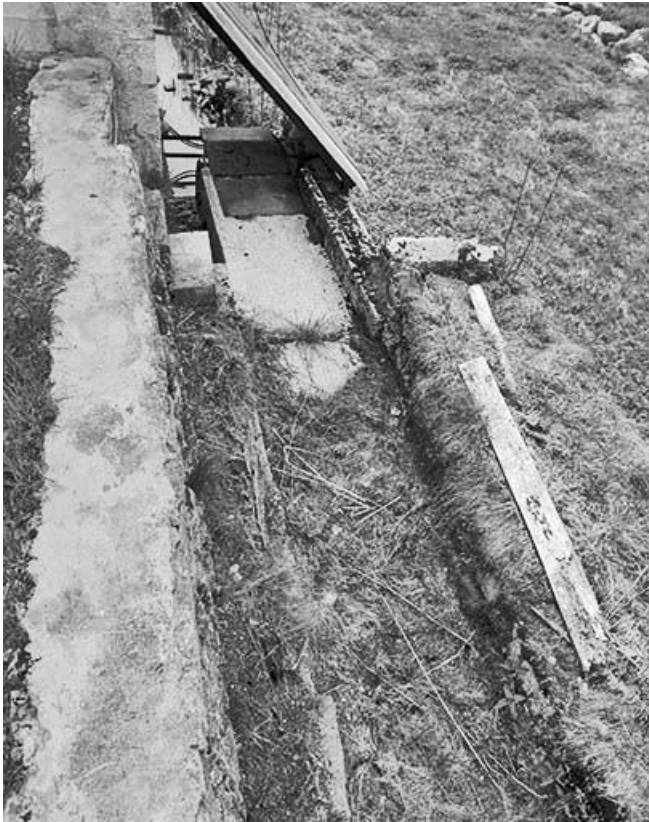
Canal d'amenée d'eau sur la roue ou " arivoir " . 39, Longchaumois, lieudit : les Moulins Piquands
